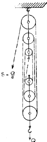
Č. 2208. Kladkostroj násobný.
