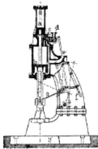
Č. 2199. Reineckerův buchar.
