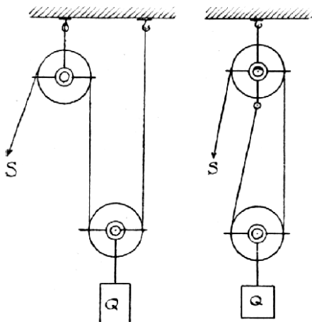
Č. 2205. a 2206. Spojení kladky hybné s nehybnou.
