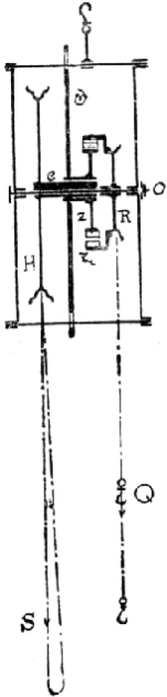
Č. 221. Eadův kladkostroj epicykloidní.
