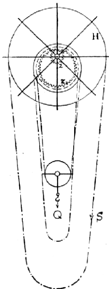
Č. 2210. Kladkostroj diferenciální s Tangyevým převodem.
