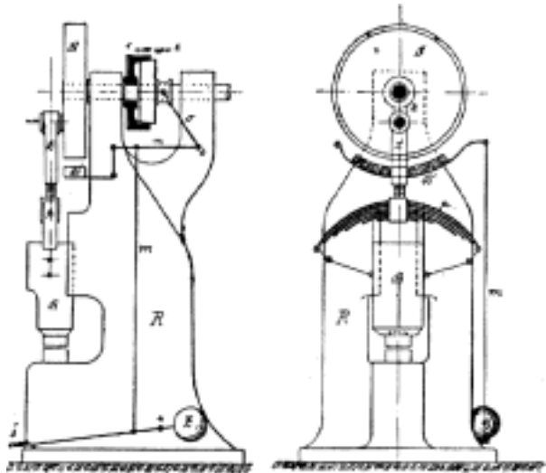
Č. 2195. Buchar perový.
