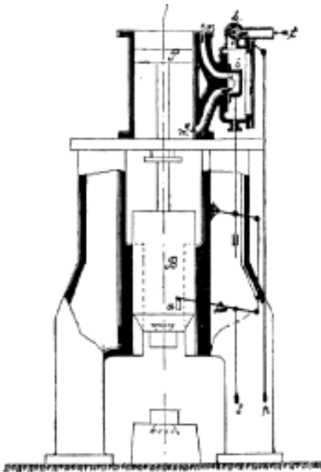
Č. 2198. Nasmythův buchar.
