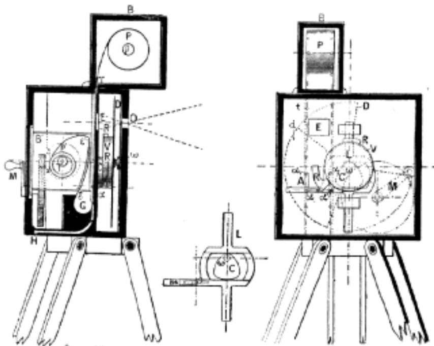
Č. 2188. Kiné matograf. Řez podélný Řez příčný
