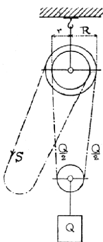
Č. 2209. Westonův kladkostroj diferenciální.
