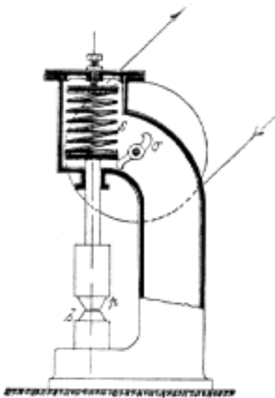
Č. 2194. Procterův buchar.
