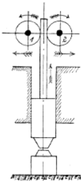
Č. 2197. Frikční buchar.
