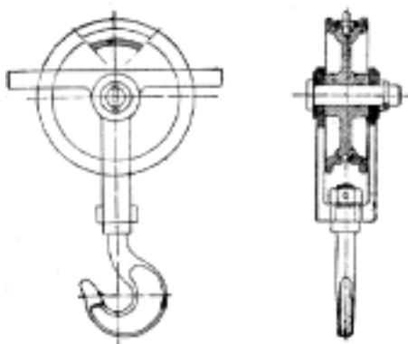
Č. 2201. Kladka řetězová.
