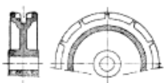
Č. 2202. Ozubená kladka řetězová.
