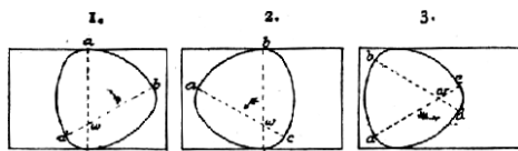
Č. 2189. Různé polohy trojúhelníka.
