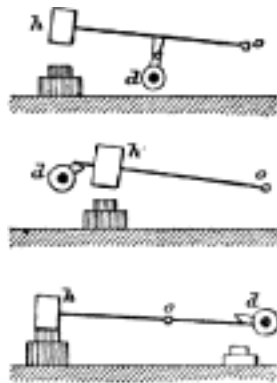
Č. 2193. Buchar: nadhazovaný, čelní, stlačovaný.
