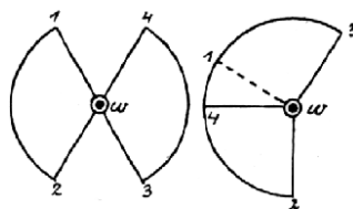
Č. 2190. Segmenty kruhové.
