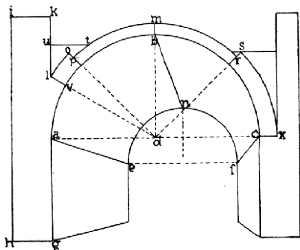
Č. 2234. Klenba a její součástky.
