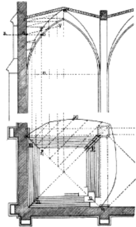
Č. 2241. Klenba křížová stoupající.
