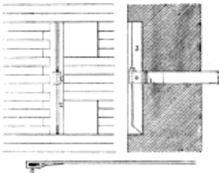
Č. 2259. Kleště do zdi.
