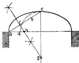
Č. 2248. Ellipsový oblouk 60tistupňový.
