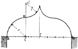
Č. 2255. Oblouk španělský č. oslí hřbet.
