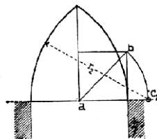
Č. 2252. Gotický oblouk z doby úpadku.
