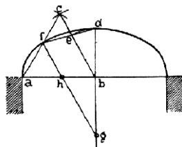
Č. 2247. Ellipsový oblouk 60tistupňový.
