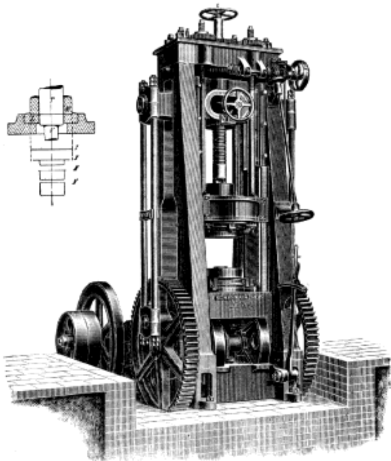
Č. 2233. Průhon s pohyblivým stolem a pevným upínadlem.
