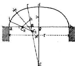
Č. 2249. Ellipsový oblouk opsaný z 5 středů bodů.
