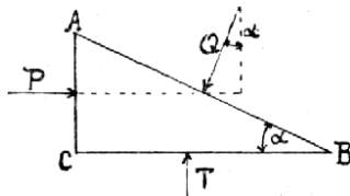
Č. 2269. Klín jednoduchý
