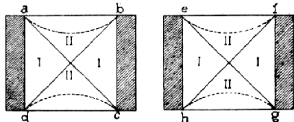
Č. 2235. Odvojení klenby klášterní a křížové z klenby valené.
