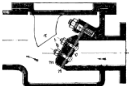
Č. 2217. Klapka kožená.
