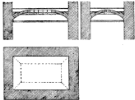
Č. 2238. Napodobená klenba zrcadlová.
