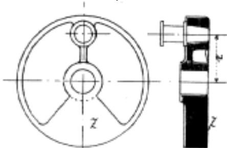
Č. 2268. Klikový kotouč.
