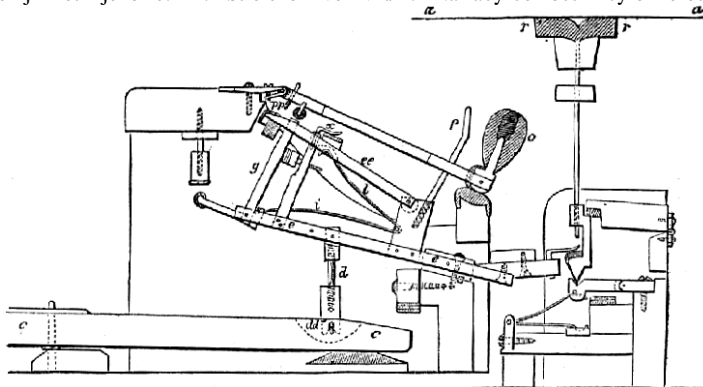
Č. 2226. Mechanika repetiční (anglická). c kláves; d sloupek, jenž lomenou pákou eg vyvrst'uje kladívko o; páka ee, jejíž zdvižení zadržováno jest při pp, způsobuje při x druhé vyšinutí pomocí pružného pera il (dvojité spruhy) i tehdy, nebyl-li kláves zcela vrácen do klidu; p chytáč; r dusítko, vlivem klávesu tlačené dolů pod strunu a, na níž v klidu jest položen.
