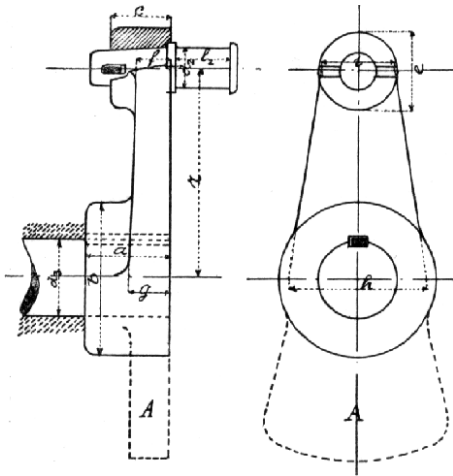
Č. 2266. Klika strojová.
