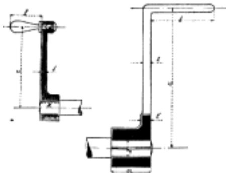
Č. 2265. Kliša ruční.
