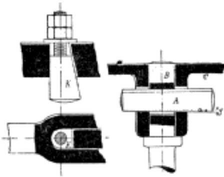
Č. 2271. Klín stavěcí.
