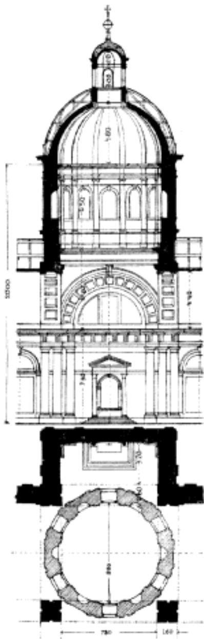
Č. 2239. Klenba baňová na tambouru, spočívajícím na pendenteích.
