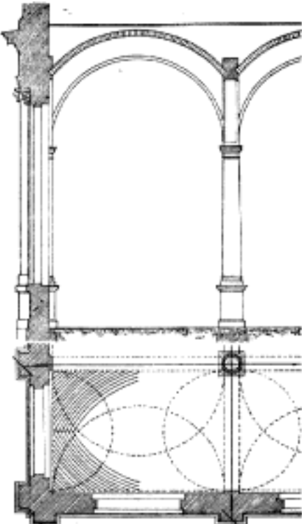
Č. 2240. Klenba česká čili česká placka.
