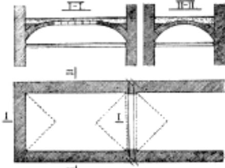
Č. 2237. Klenba neckovitá.
