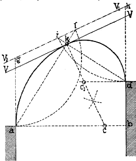
Č. 2288. Sestrojení kobyli hlavy, kde dány jsou obě patky a směr tečny.
