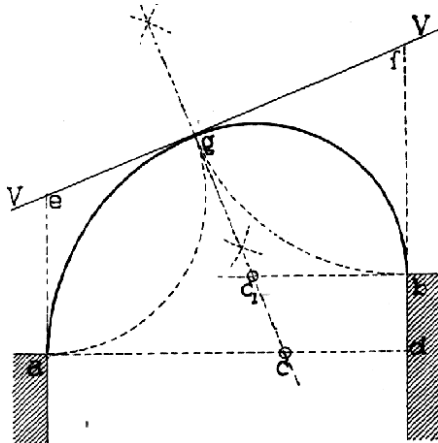
Č. 2287. Sestrojení kobyli hlavy, kde dána jest jedna patka a tečna k ní.
