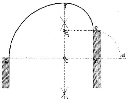
Č. 2285. Kobyli hlava sestrojena ze dvou kvadrantů.
