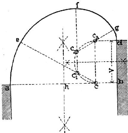
Č. 2286. Kobyli hlava sestrojena ze čtyř částí kružnice.
