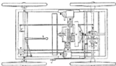
Č. 2293. Motorový kočár Gauthier-Wehrléův.
