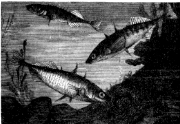
Č. 2297. Koliška obecná ( Gasterosteus aculeatus L.).
