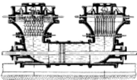
Č. 2308. Mokrý kompressor Hanarteův.
