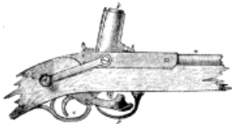
Č. 2303. Norská komorovka z r. 1842. a hlavě, k komora, z zápalník, m kohoutek, p zpruha, s spoušť, d klíka.
