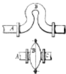
Č. 2304. Kompensátor při potrubí.
