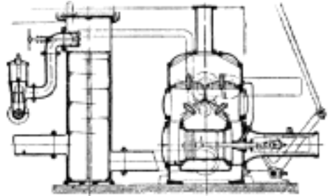
Č. 2312. Kondenzátor s vývěvou soustavy L. A. Riedingera.
