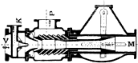
Č. 2310. Kondenzátor Körtigův.
