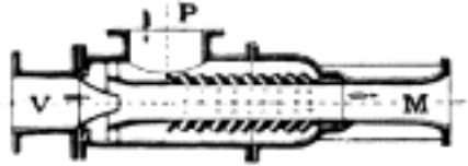
Č. 2311. Kondenzátor Körtigův.
