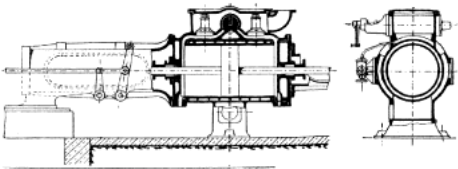
Č. 2307. Suchý kompressor Harrasův.
