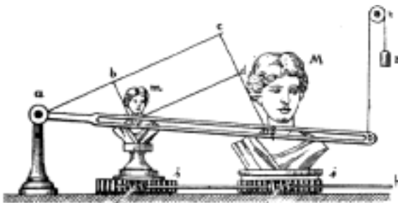
Č. 2316. Přístroj ku kopírování soch.
