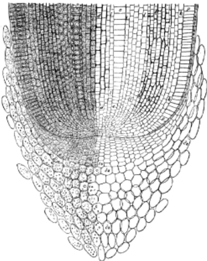
Č. 2317. Podélný řez kořenem rostliny jevnosnubné (kukuřice, Zea mais ), č. zevnější starší vrstvy čepičky, č. vnitřní mladší její vrstvy; v bod vrcholový; d e l pleroma, d budoucí dřev, c céva, l dřev, x k kůra z periblamu pocházející, p pokožka se stlupými vnějšími stěnami. Toliko v levé polovině naznačen obsah plasmový a jádra v buňkách.
