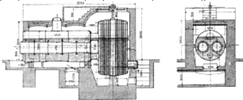
Č. 2333. Kotel Dupuisův.
