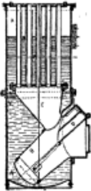
Č. 2336. Stojatý kotel s Tenbrinkovým topením.
