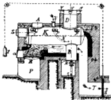
Č. 2328. Jednoduchý kotel válcový.
