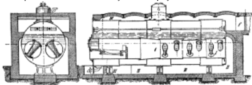
Č. 2331. Lancashirský kotel s Gallowayovými rourami.
