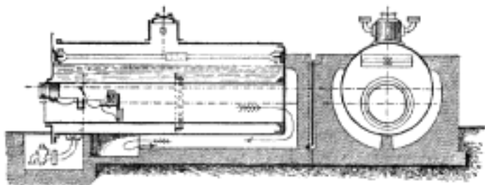
Č. 2330. Cornwallský kotel.
