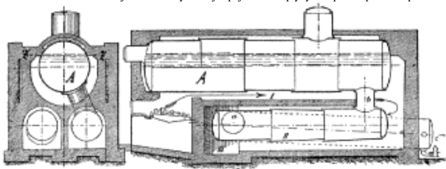
Č. 2329. Kotel se dvěma zpodníky.
