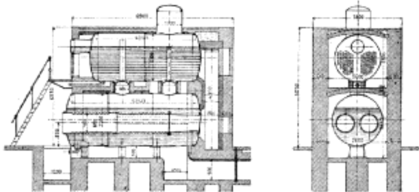
Č. 2335. Kotel Tischbeinův.
