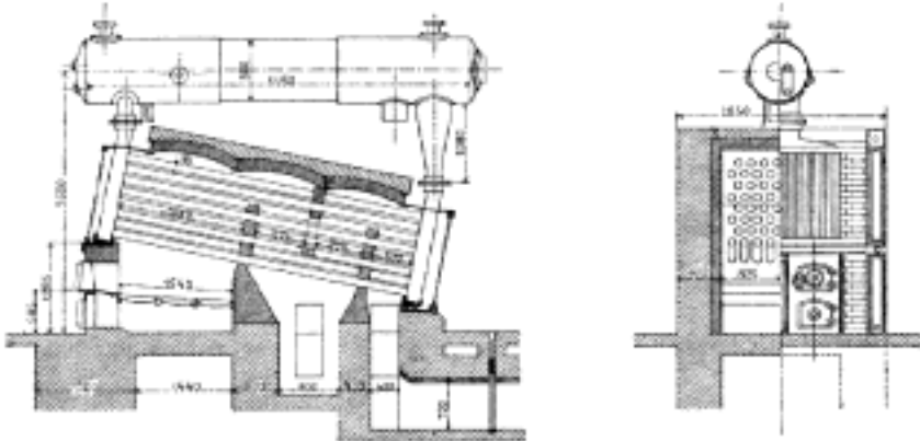
Č. 2332. Kotel Steinmüllerův.
