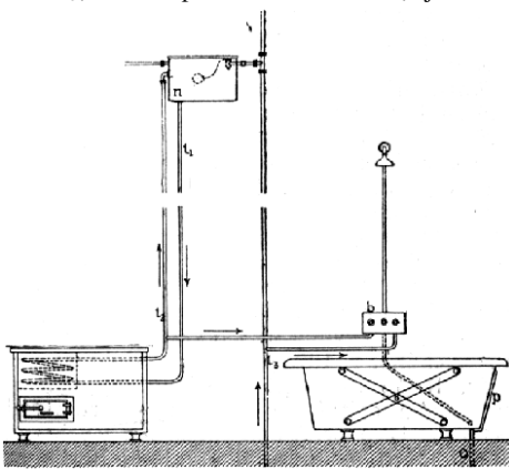
Č. 2345. Zařízení koupelny, kde voda se ohřívá v kuchyňském sporáku.
