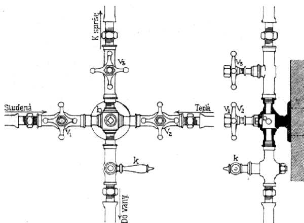
Č. 2343. Směšovací batterie, kde studená i teplá voda jest pod tlakem.
