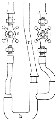
Č. 2342. Směšovací baterie pro vodu studenou a teplou pod tlakem se nacházející.
