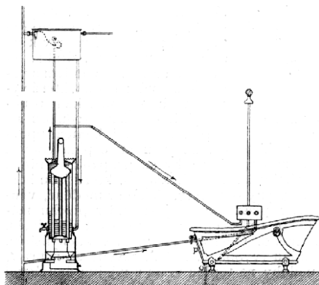
Č. 2346. Zařízení koupelny, kde voda se ohřívá v lázeňských kamnech.
