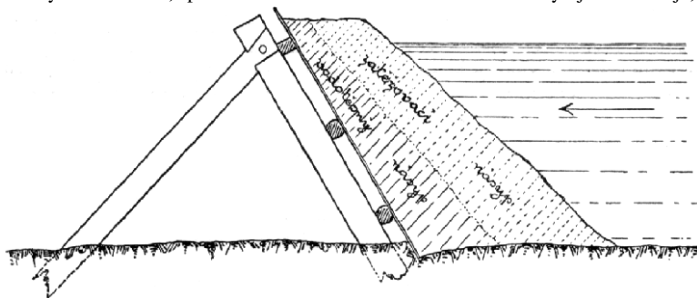
Č. 2358. Koz pro jímku.
