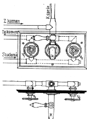
Č. 2344. Směšovací batterie, kde teplá voda není pod tlakem.
