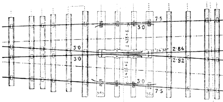
Č. 2385. Křížovatka ostroúhelná, neúplná.
