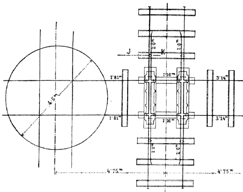
Č. 2383. Křížovatka pravouhelná.
