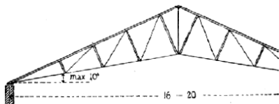
Č. 2404. Profil krovu soustavy německé.
