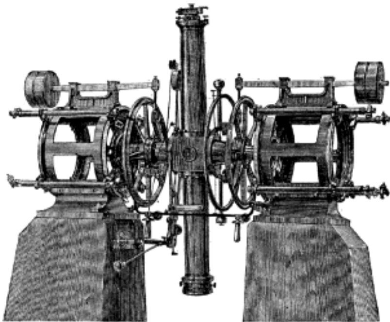
Č. 2407. Repsoldův kruh poledníkový.
