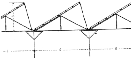
Č. 2399. Profil střechy shedové.
