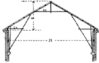
Č. 2400. Profil krovu soustavy Ardantovy.
