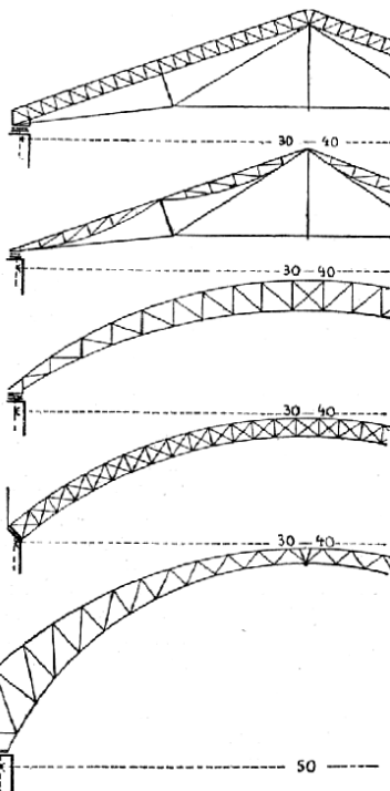
Č. 2405. Profily železných krovů velikého rozpětí.
