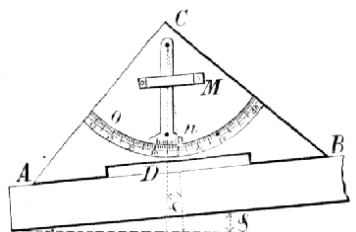
Č. 2389. Krokvace hornická.
