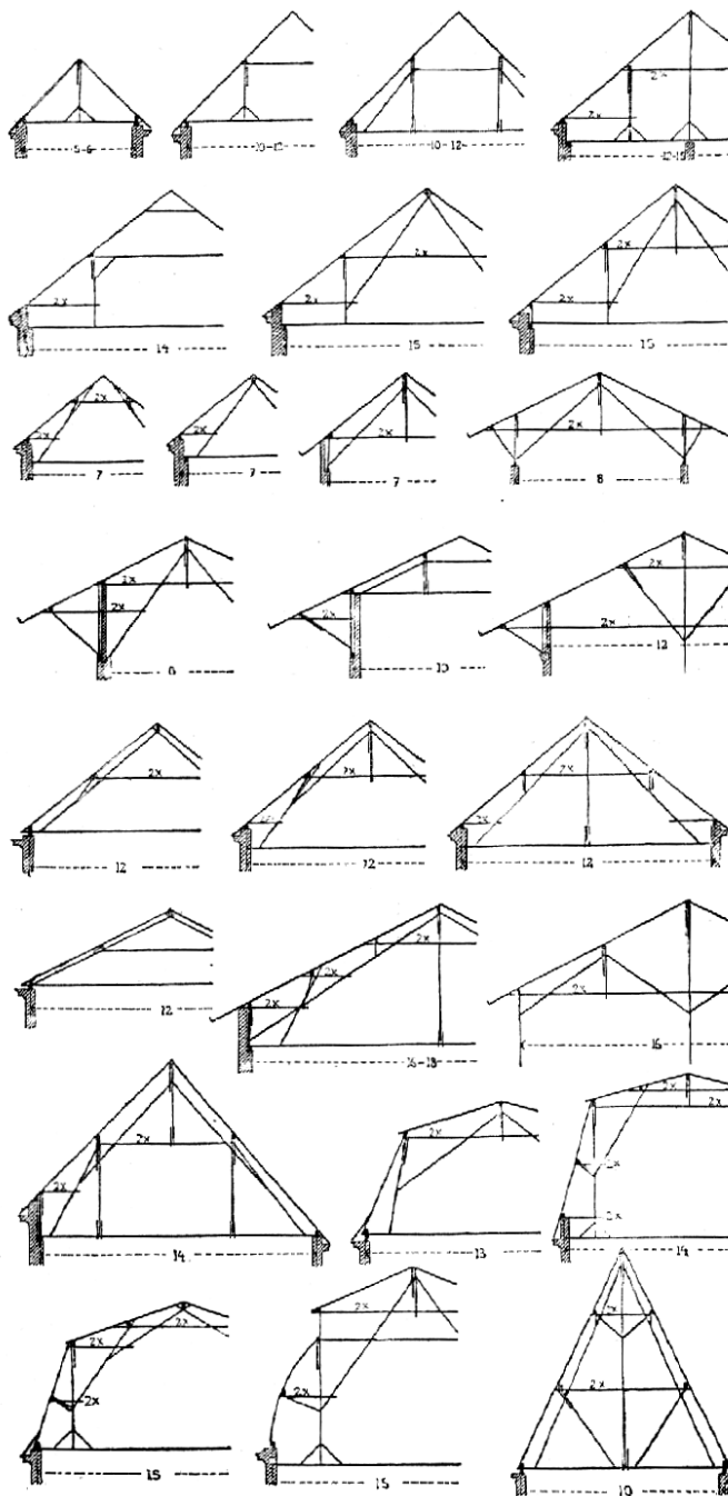
Č. 2397. Profily plných vazeb soustavy vaznicové.
