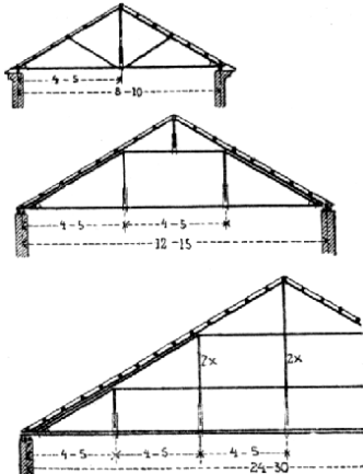
Č. 2398. Profily krovů soustavy vlaské.
