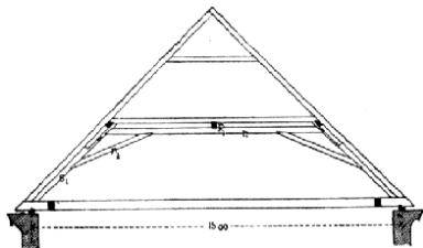
Č. 2396. Profil ležaté stolice německé.
