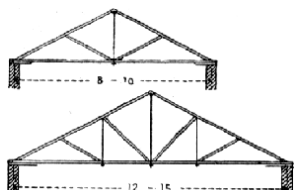
Č. 2402. Profily krovů soustavy anglické.
