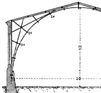
Č. 2401. Profil krovu soustavy vzkružové.
