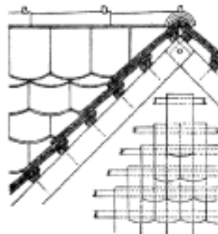
Č. 2416. Dvojnásobná tašková krytina na husté laťování.
