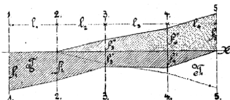
Č. 2432. Kubatura: způsob přibližný.
