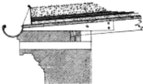
Č. 2427. Krytina z dřevitého cementu.
