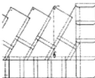
Č. 2419. Jednoduchá krytina břidlicová.
