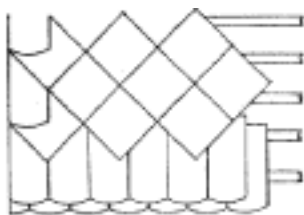
Č. 2417. Jednoduchá krytina čtvercovými taškami.
