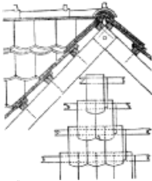
Č. 2414. Jednoduchá tašková krytina na louč.
