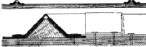
Č. 2428. Krytina lepenkou svitkovou.
