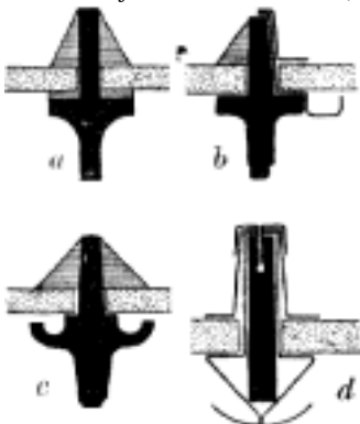
Č. 2429. Železná žebra pro krytinu skleněnou.
