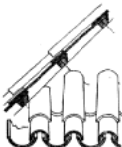
Č. 2418. Krytina rúrková.
