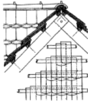
Č. 2415. Dvojnásobná tašková krytina t. zv. korunová.
