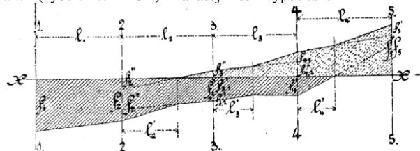
Č. 2431. Kubatura: způsob prakticky určitý.
