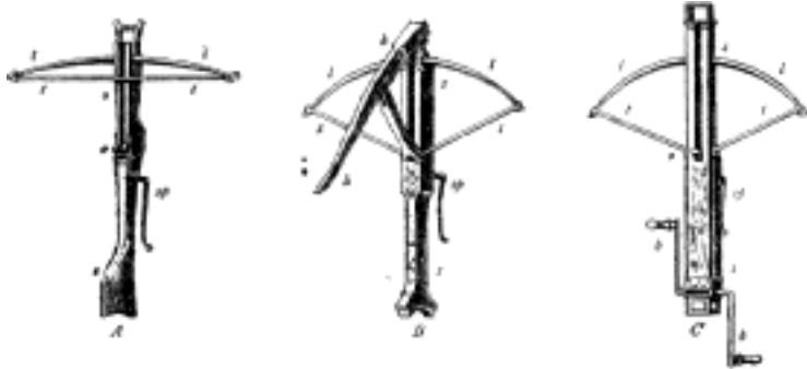
Č. 2440. Kuše. A) Kuše s lukem nenapjatým. B) Kuše s lukem napjatým pomocí heveru. C) Kuše s lukem napjatým klikou. s socha, l luk, t tětiva, o ořech, sp spoušť, h hever, k klika.
