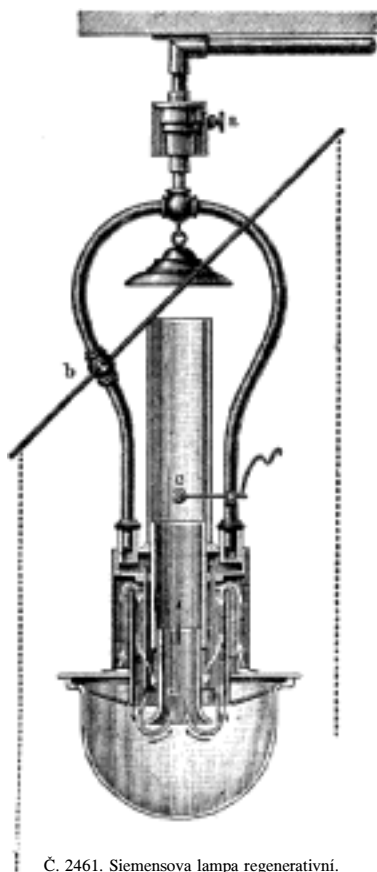
Č. 2461. Siemensova lampa regenerativní.
