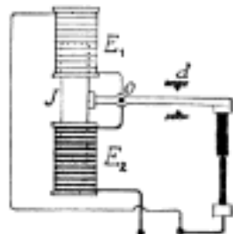
Č. 2469. Schéma lampy diferenciální.
