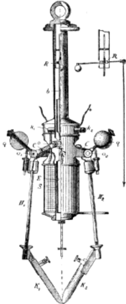
Č. 2475. Lampa Schleyderova.
