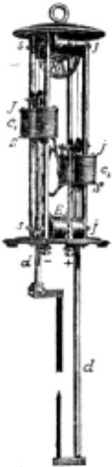
Č. 2474. Lampa Doubrava-Donátova.
