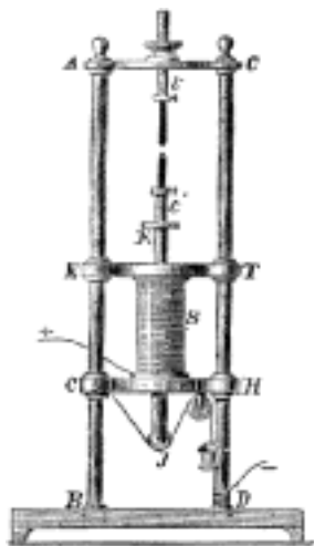
Č. 2465. Archereauův regulátor.
