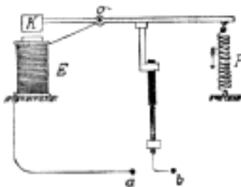
Č. 2467. Schéma lampy seriové.
