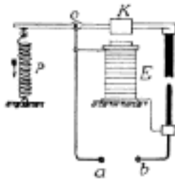
Č. 2468. Schéma lampy derivační.
