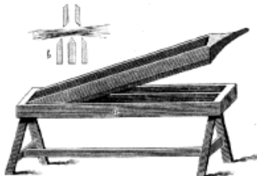
Č. 2491. Trdlíce: a se strany, b průřez.
