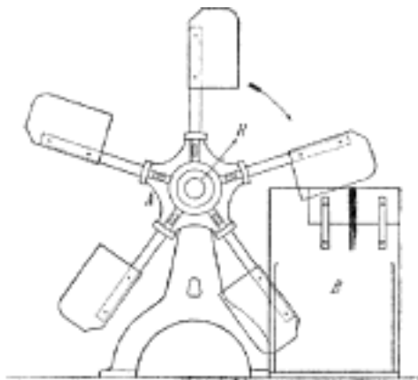
Č. 2499. Stroj potěrací.
