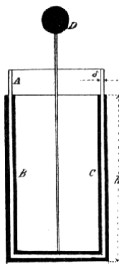
Č. 2487. Lejdská láhev.
