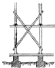
Č. 2504. Lešení pro stavbu dlouhotrvající.
