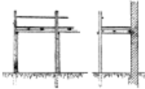
Č. 2503. Pražský způsob lešení.
