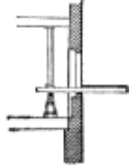
Č. 2506. Lešení vysuté.
