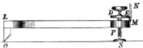
Č. 2524. Pravítko rektifikační.
