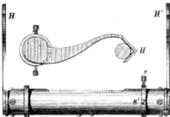
Č. 2521. Libella závěsná.
