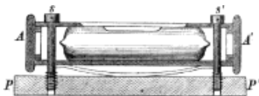
Č. 2518. Uložení skleněné trubice libell.
