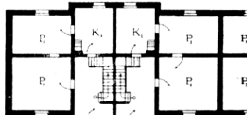
Obr 3. Obytné domy f ve Vítkovicích o 16 bytch
