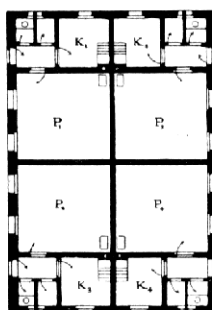
Obr.7. Přízemní domek o 4 bytech akc. spol. Hrástky a Prádelny na Smíchově
