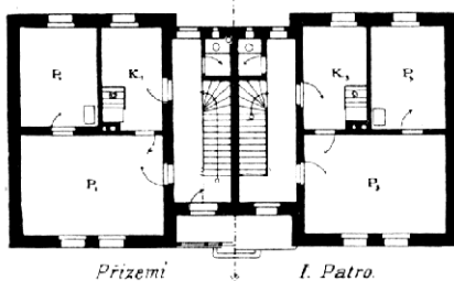
Přízemí I. Patro
