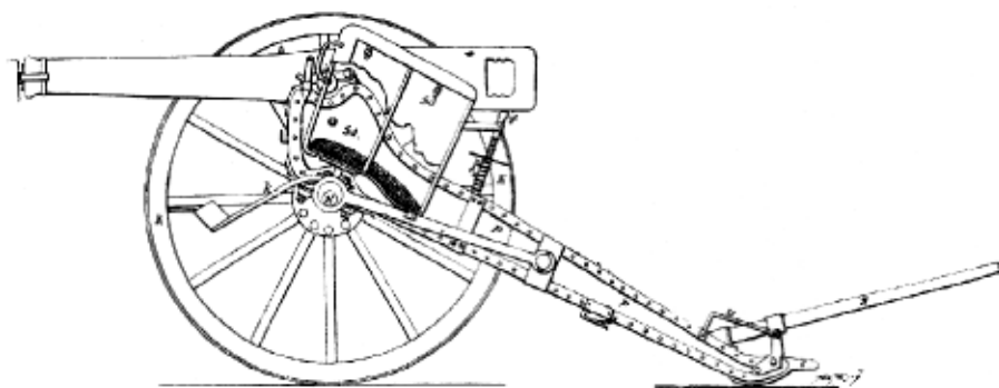
\frac{1}{48} Rakouské (vz. z r. 1875) odhlomozené ke střelbě. K kolo, P postranice lafety, Sd sedadlo, F řidičlo, N náprava, u ucho u zadku lafety, c zadek lafety u kruhem, S sochor hlomozní čili řidič.
