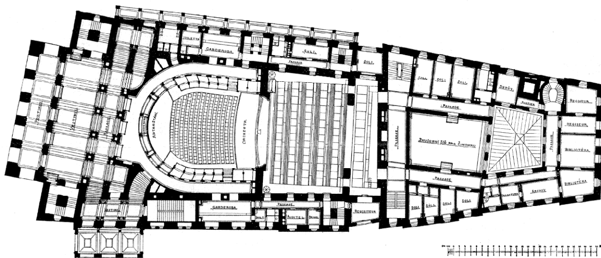
Pūdorys přízemí.
