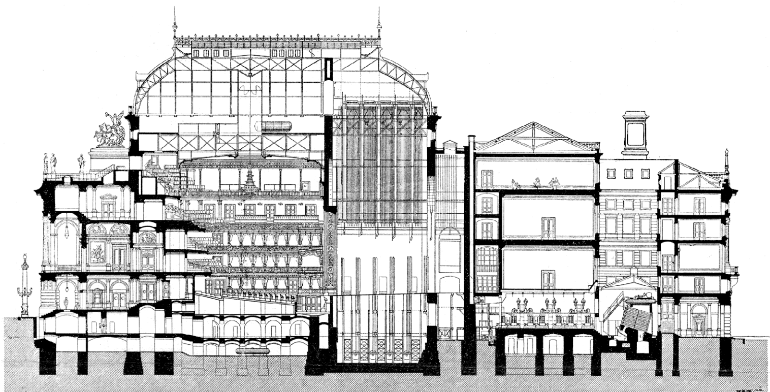
Kolmý průřez.
