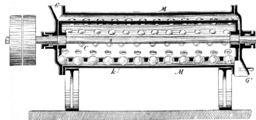
4. Hauctinovo drtidlo kulové.
