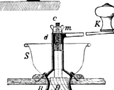
3. Konický mlýnec na kávu.
