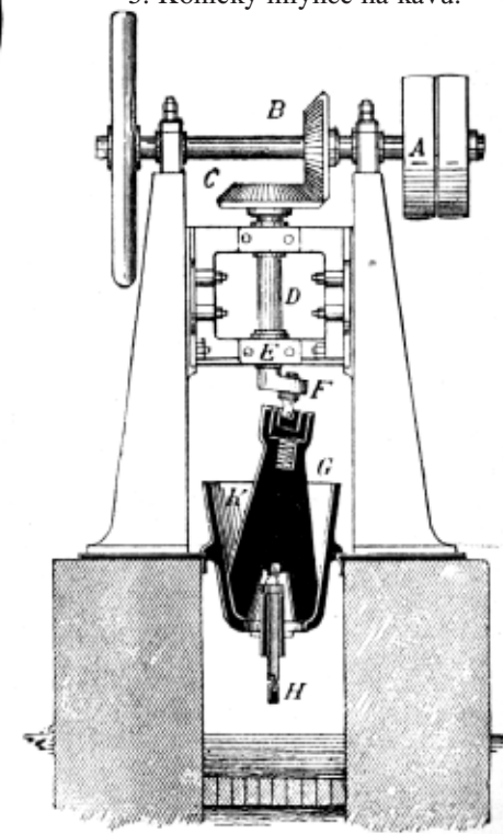
2. Renettův hmoždířový mlýnec.
