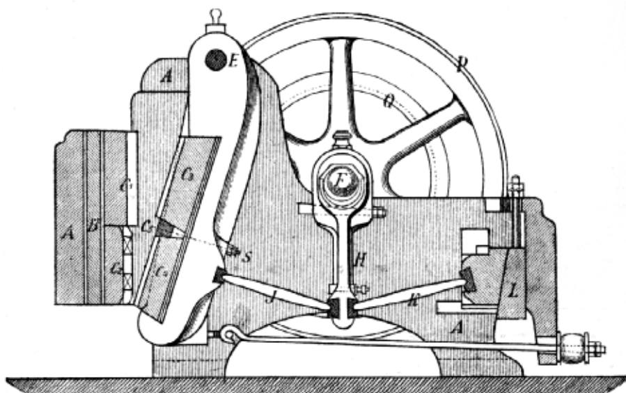
7. Blakeovo drtidlo čelistové.
