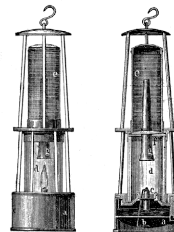
8. Mueseleroва bezpečná lampa. (věterka).
