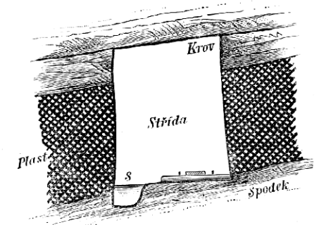
6. a 7. Průřez stříd.
