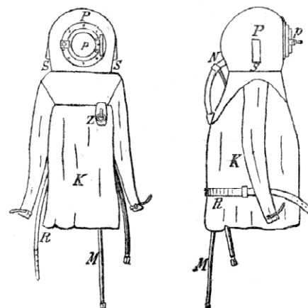
10. Zmáhací přístroj Bremenův.
