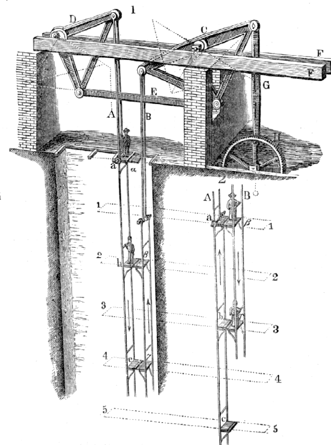
7. Lezný stroj.
