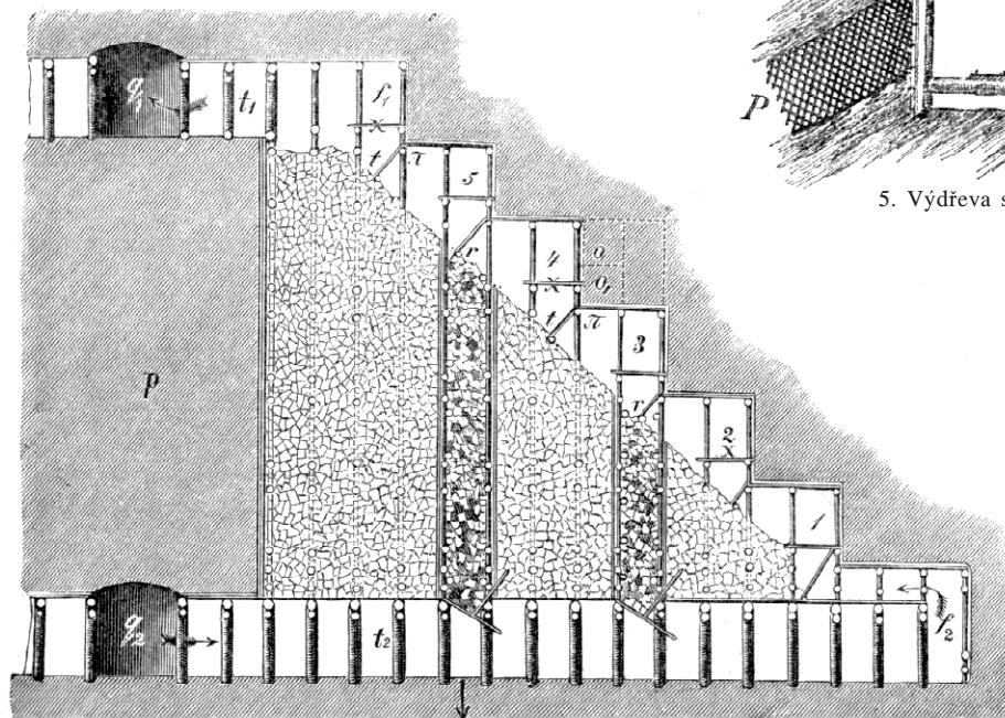
3. Dobývání výstupnými stěnami.
