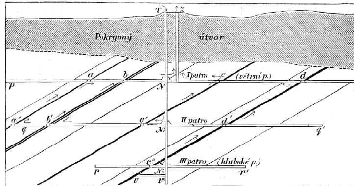
4. Průřez uhelného dolu.
