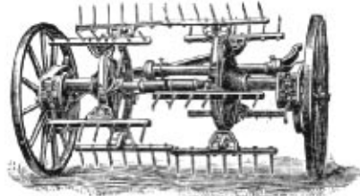
5. Stroj k obracení a rozmetávání sena.
