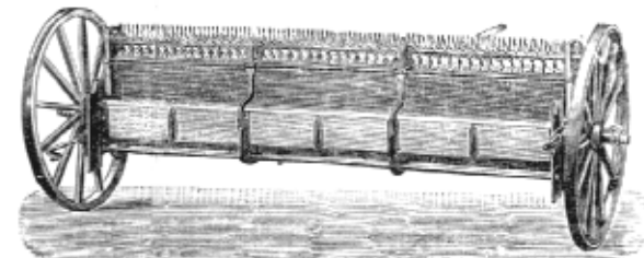
11. Schloerovo rozmetadlo hnojiva.
