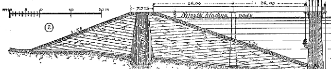
HRÁZ NÁDRŽE VODÁRENSKÉ V BOMBAY-1
