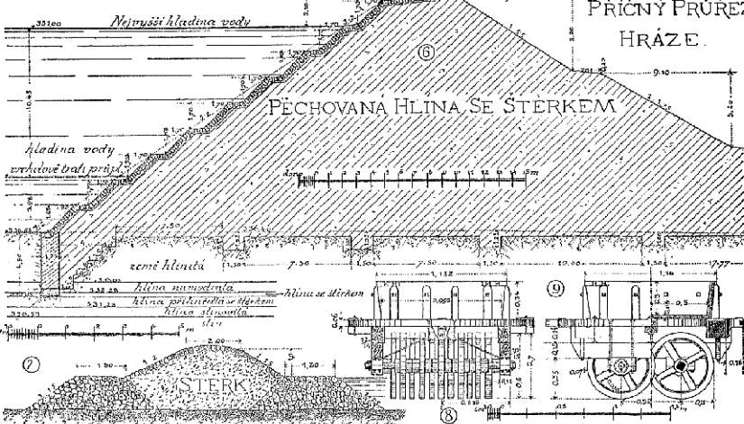
HRÁZ ŠOUSTŘEDOVACÍ NAVLTAVĚ
