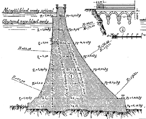
HRÁZ SAINT ÉTIENNE-SKÁ
