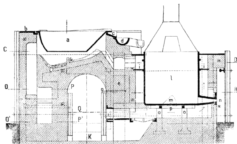
Čermákův apparát k pattinování parou (Příbram).
