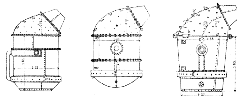
Druhy konvertrů.
