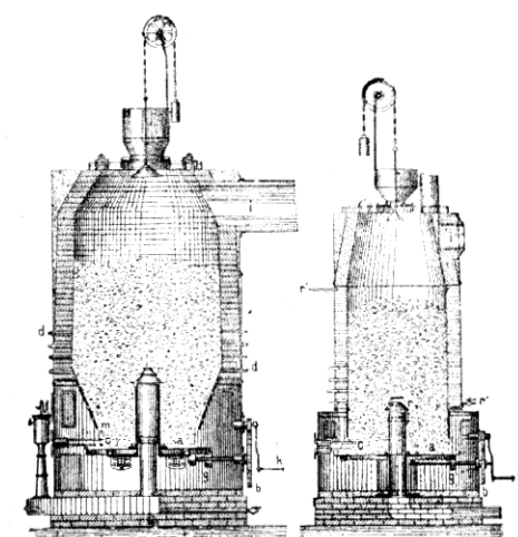
Taylorův generator.
