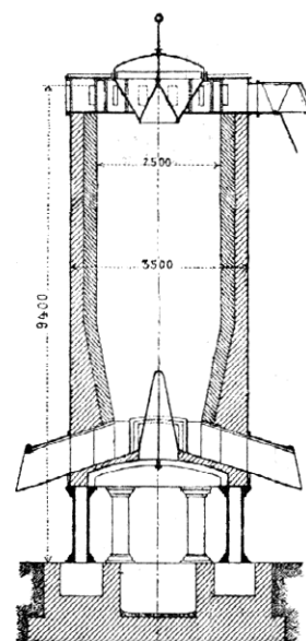
Novákova vysoká pec pražecí a kalcinační (Idrija).
