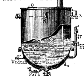
UZAVŘENÝ SATURATEUR
