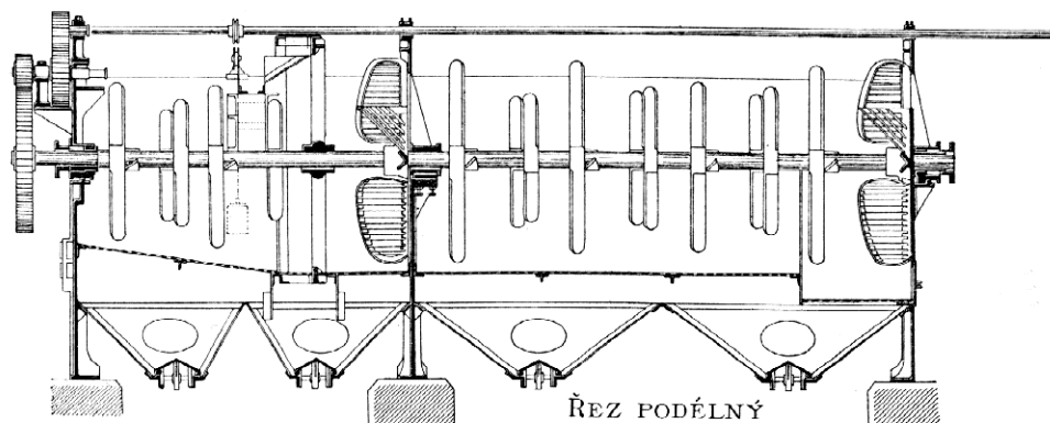
HŘEBLOVÁ PRAČKA WIESNEROVA
