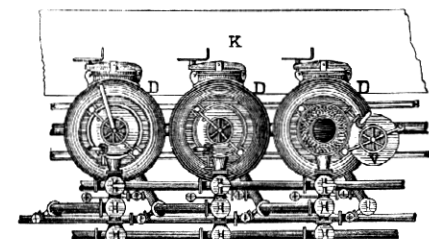
PŮDORYS DIFFUSEURŮ A SOUTRUBÍ
