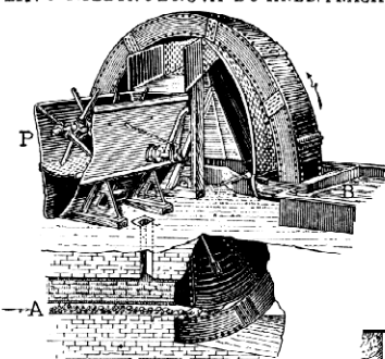
KOLO NA ZVEDÁNÍ ŘEPA ZE SPLAVU RIEDINGEROVA DO HŘEB. PRAČKY
