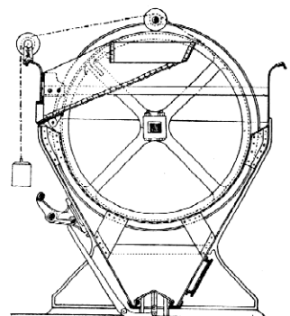
ŘEZ PŘÍČNÝ
