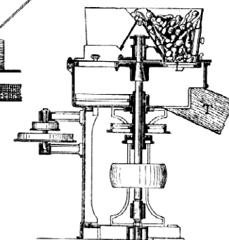
ŘEZAČKA NA ŘEPU
