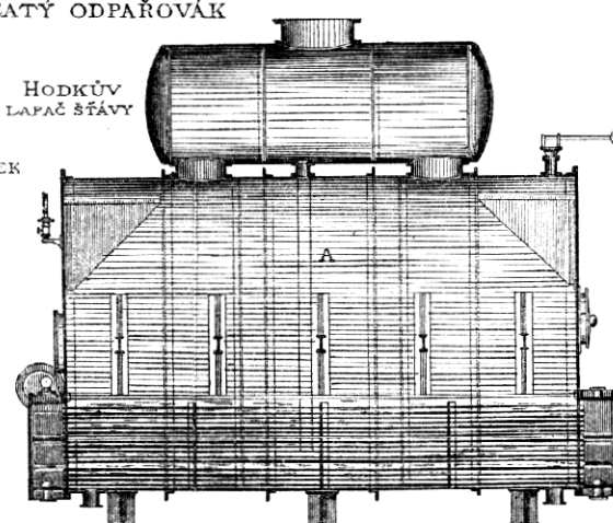
POHLED
