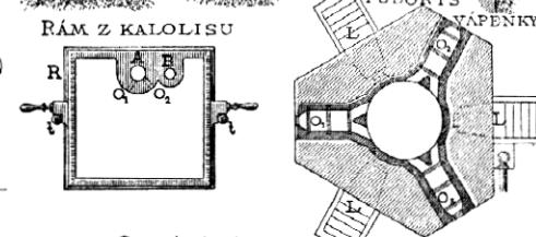
PŮDORYS VÁPENKY
