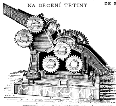
PĚTIVÁLCOVÝ MLÝN NA DRCENÍ TRTINY
