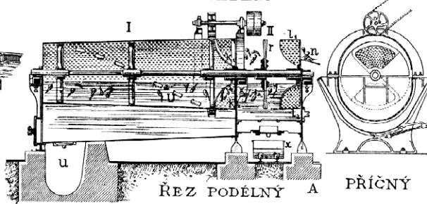
HŘEBLOVÁ PRAČKA WIESNEROVA
