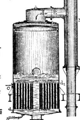
STÁVA PRŮLEH K UČISTĚNÍ
