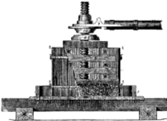
Č. 2538. Lis šroubový dle rýnského způsobu.
