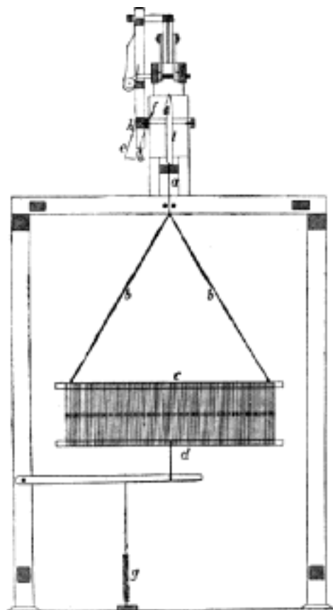
Č. 2556. Ruční listový stroj.
