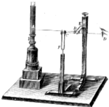
Č. 2545. Přístroj pro vyvozování Lissajousových křivek.
