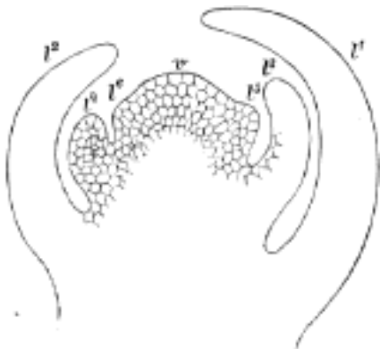
Č. 2551. Podélný řez vrcholkem stonku v s listy l-l' - 16.
