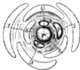
Č. 2552. Pohled na vrcholek v stonku a listy dle 2/5, 1-6 listů odříznuté. 7-9 nejmladší celé hrbolky listové.
