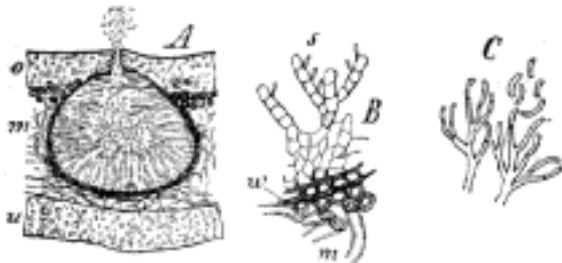
Č. 2563. A Spermatogonium čili pyknida lišejníku Gyrophora cylindrica (L.) Ach. v optickém, kolmém průřezu. Nádržka ponoření ve stélce jest uložena ve dřeni m a zasahá svým temenem do svrchní kory o, kterouž poněkud nadzvedla a malým otvorem prorazila. Z něho něco spermií vytrysklo; u spodní vrstva korová stélky. Zvětš. 90krát dle De Baryho. - B Malý kousek vnitru téhož spermatogonia, v stěna jeho s přiléhajícími vláknými dřevinami vrstvy m; s sterigmata článkovaná, arthrosterigmata se spermiemi. Zvětš. 390krát dle De Baryho. - C Rozvětvená sterigmata a rohličkovité spermiace lišejníku Cladonia Novae Angliae Del. Zvětš. 450krát dle Tulasnea.
