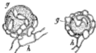
Č. 2566. Řasa Protococcus ( Cystococcus ) g, chromidie ze stélky lišejníku Cladonia furcata (Huck.), Fr., opředené houbovými vlákny h těsně k povrchu řasy přiléhajícími. Zvětš. 959krát dle Borneta.
