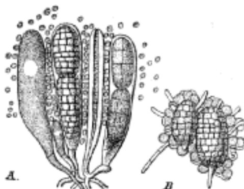
Č. 2567. A Část hymenia z kolmého průřezu plodu lišejníku Endocarpon pusillum Hedw. s několika větví dvouvýtrusými, mezi nimiž volně uloženo jest množství hymeniálních gonidií. B Dva mnohohlodné výtrusy téhož lišejníku, vyvrstvené z větve, se lpějícími na nich hym. gonid., jež obemknuty vyražejícími klíčními vlákný se zvětšily (povyostly).
