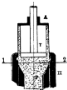
Č. 2543. Lisování hrců.
