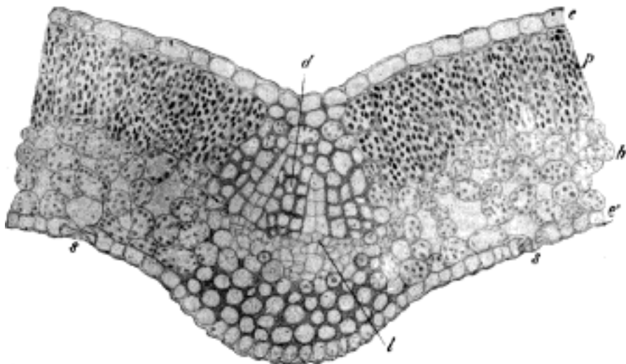
Č. 2554. Anatomický průřez listem ptačího zobu japonského ( Ligustrum lucidum Hort.).
