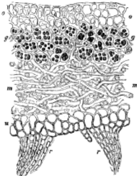
Č. 2558. Kolmý průřez chrástovitou stélkou Stictia fuliginosa (Dicks.) Nyl. Svrchní kora o a a spodní kora u ukazují velmi dobře velikou světlost (lumen), průměr buněk houbových, těsně k sobě narostlých. Při r vidíme rhizoidy v podélném průřezu; g vrstva chromidiová, sestávající z buněk řasy Chroococcus , obalených tlustou, bezbarvou blanou rosolovitou; m vrstva dřevná z vláken volně propletených složená. Zvětšeno 500krát dle Sachsa.
