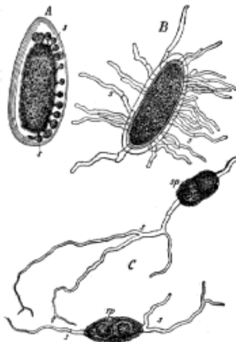
Č. 2562. Klíčící výtrusy lišejníků. A Jednoduchý, veliký výtrus lišejníku Pertusaria communis DC. po 24hodiněm bobtnání v glycerinu, s začátky klíčících vláken vchlípují se do endosporia. B Podobný výtrus lišejníku Pertusaria leioplaca (Ach.) Schaer., kde vyrostla vlákna klíční proražením exosporia na venek. Zvětš. 310krát dle De Baryho. C Výtrusy dvoubuněčné sp lišejníku Solorina saccata (L.) Ach. s povyroslými a leckde již rozvětvenými klíčními vlákny s, vždy po jednom z každého dílu výtrusového. Zvětš. 270krát dle Tulasnea.
