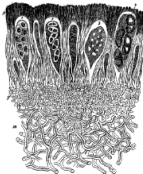
Č. 2561. Malý kousek kolmého průřezu zralou plodnicí lišejníku Anaptychia ciliaris (L.) Kbr., p rouško složené z vláken podpůrných, parafys, a z vřecek, mezi předešlé vsunutých. Č. 1. - 4. vyznačuje postupný vývoj výtrusů vřecku. Nečíslovaná, uzounká a kratší vřecka jsou nejmladší. Č. 4. představuje vřecko s výtrusy dokonale vyvinutými, hnědými a dvoudílnými, y vrstva podroušková, m vrstva dřevná. Zvětš. 440krát dle Sachsa.
