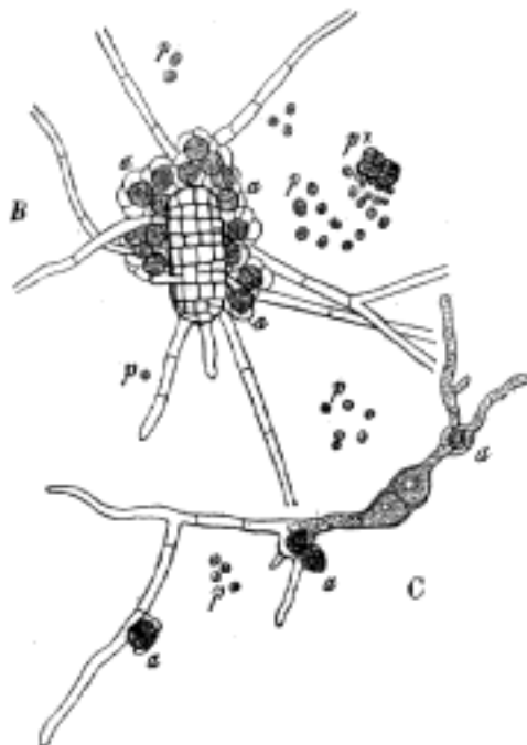
Č. 2568. B Starší stadium klíčnímu výtrusu lišejníku Endocarpon pusillum Hedw. Hymeniální gonidie a jsou tu již dokonale opletena klíčními vlákný, která se také tu a tam prodloužila a rozvětvila; p volné hymen. gonid., nezměněné; px hym. gonid. zakládající kolonii normálně řasy Pleurococcus . C Klíční, dvoudílný výtrus lišejníku Thelidium minutulum Körb. (stálého to souseda lišejníku End. pusillum ), jehož klíční vlákná obemkla také hym. gonid. a, pocházející z lišejníku End. pusillum ; p ještě volné hym. gonid. Zvětš. 320krát dle reprodukce Fünfstückovy (Pflanzenamilien) podle Stahla.
