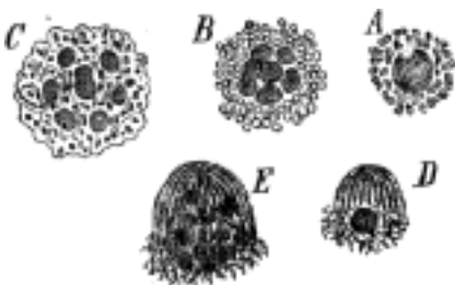
Č. 2559. Sorediové částice lišejníku Usnea barbata Fr. v opt. průřezu. A Volný soroblast, jediná buňka řasová (cystococcus) opletená vláknou houbovou. B Soroblast, jehož buňka řasová rozdělila se ve více buněk. C Soredula povstala z volného soroblastu oddálením pomnožených buněk řasových, jež znovu vlákna houbová obrostla. D Volný soroblast zakládající novou stélku; E též v pokročilejším stupni vývoje. Zvětš. asi 500krát. Dle Schwendenera.
