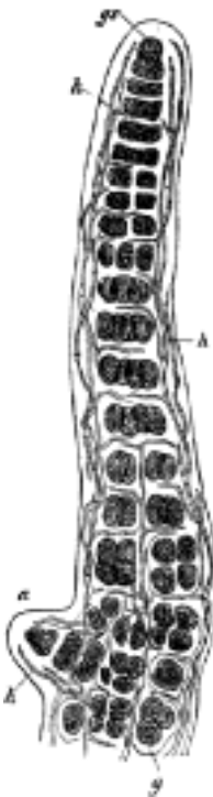
Č. 2557. Vlákenná větvička stélková lišejníku Ephebe pubescens Fr. s počátkem nové mladší větvičky při a (v optickém průřezu). Uvnitř obou větví jsou umístěny rozestouplé chromidie, t. j. buňky řasy Sirospion G., jichž rosolovitě blány prorostla vlákna houbová, hyfy h. Jednoduché vlákno řasové v původním stavu vidíme ještě na koncích obou větví: při gs, potom při a, kde také vlákna houbová ještě se nerozvětřila. (Zvětš. 5000krát. Dle Sachsa.)
