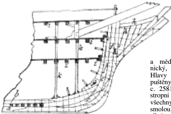
Č. 2576. a kýl, b vnitřní kýl, c vnitřní přední stěven, f přední stěven, g klec pro přední stěven, h výplňová dřeva gallionu, i trámce podpalubní, k sloupky ku podpore palub.
