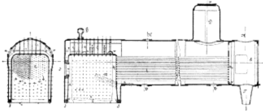
Č. 2605. a 2606. Kotel lokomotivní : průřez příčný a podélný (skrácený).
