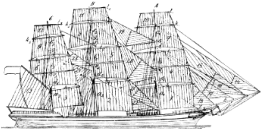
Č. 2588. A Přední stěžen (Fockmast). B Střední stěžen (Grossmast). C Zadní stěžen (Kreuzmast, Besanmast). a1, a2, a3 spodní díly stožárů; b1, b2, b3 střední díly; c1, c2, c3 horní díly; d1, d2, d3 spodní ochozy ( Topp ); e1, e2, e3 k nim příslušné zděře ( Eselshaupt ); f1, f2, f3 horní ochozy; g1, g2, g3 zděře; h1, h2, h3 spodní rahna; i1, i2, i3 střední rahna ( Marsraa ); k1, k2, k3, l1, l2, l3 horní rahna ( Bramraa a Oberbramraa ); 1, 2, 3 spodní plachty ( Untermastseel ); 4, 5, 6 střední plachty ( Marssegel ); 7, 8, 9 a 10, 11, 12 horní plachty ( Bramsegel a Oberbramsegel ); 13 stojatá plachta ( Gaffelsegel ); D osten ( Bugsprit ); E nástavec ( Klüverbaum ); 14, 15, 16, 17, 18 trojrohé přední plachty ( Klüver ); 19, 20, 21, 22, 23, 24 trojrohé plachty mezistěžní.
