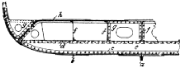
Č. 2583. a plný kýl, b vnější stěna plechová, c vnější úhelník žebra, d vnitřní úhelník, e vertikální plech spojující úhelníky, f podélná žebra, g podporné plechy, h vnitřní dno.
