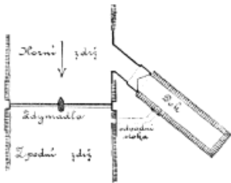
Č. 2593. Loděnice ve způsobě komorového plavidla.
