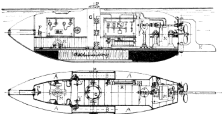
Č. 2591. Potápěcí loď »Sandor Back«.
