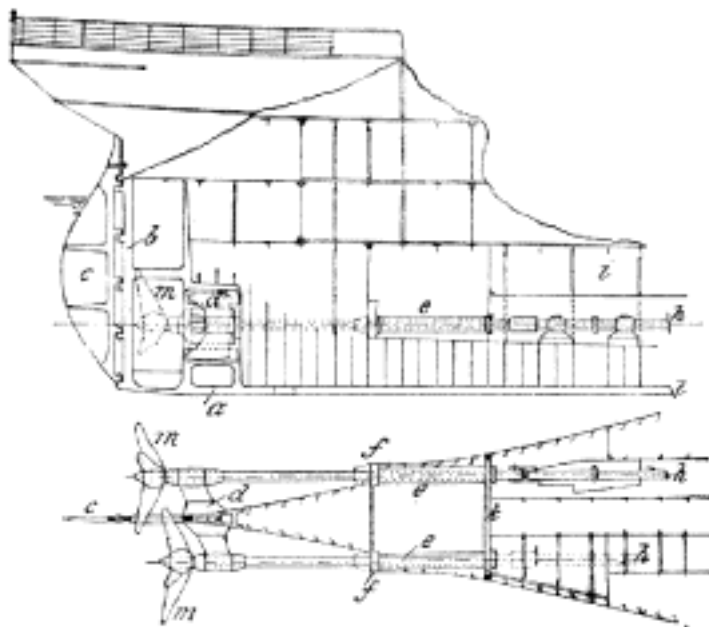
Č. 2585. a zadní steven, b steven pro kormidlo, c kormidlo, d konsoly pro hřídel, e roura hřídelová, f výstup hřídele z trupu lodi, h hřídel šroubový, i tunel pro šroub, k přehrada se zacpávkou hřídele, l kýl, m šroub.
