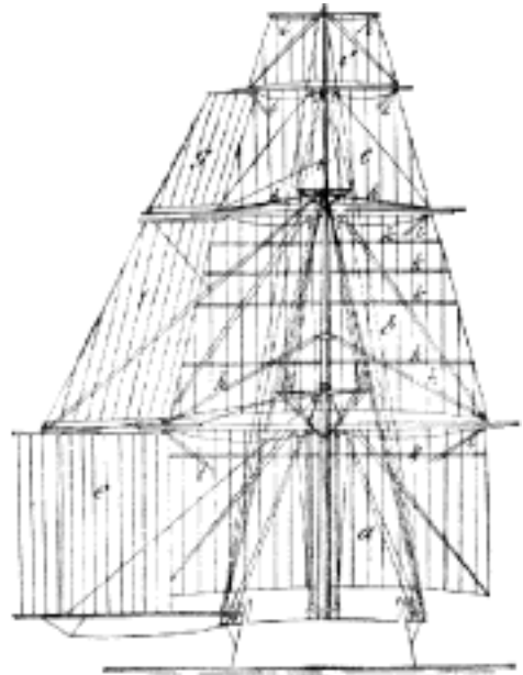
Č. 2587. Rahnové plachty: a spodní plachta ( Untersegel ), b střední plachta ( Marssegel ), c, d horní plachty ( Bramsegel a Oberbramsegel ), e, f, g postranní plachty ( Unterleeseegel , Marsleeseegel , Bramleeseegel ), h lana k závěsu rahen ( Toppenanten ), i lana k řízení a přidržování plachet ( Brassen ), k pásky k zmenšení plachet.
