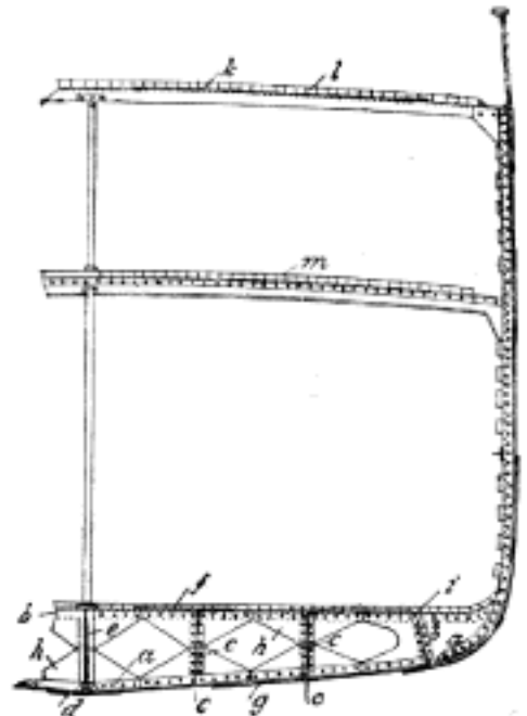
Č. 2584. a vnější úhelník, b vnitřní úhelník žebra, c podélná žebra (kýly), d střední kýl plochý, e střední kýl vnitřní, f vnitřní dno, g vnější dno, h uzlové plechy, i postranní stěna vnitřního dna, k plechové dno svrchní paluby, l svrchní paluba, m mezipaluba.
