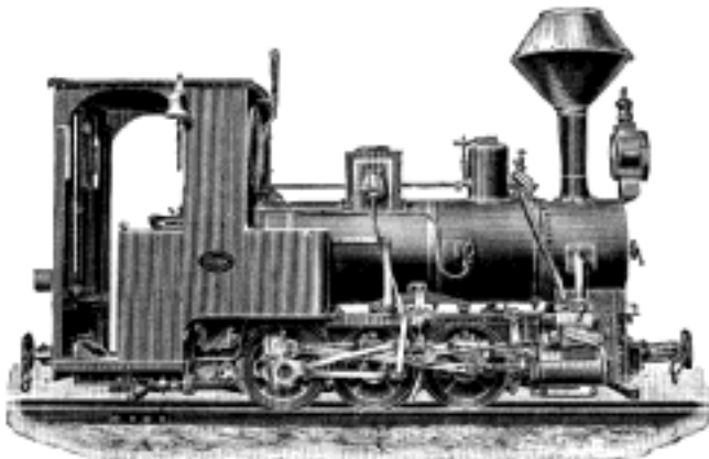
Č. 2611. Lokomotiva pro dráhy úzkokolejné s rozchodem 600 mm. Váha vystr. 86 t.
