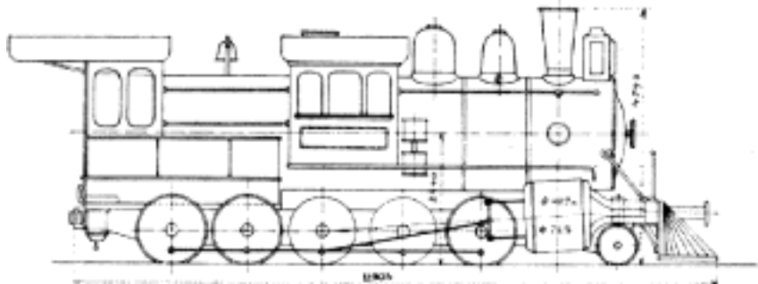
Č. 2607. Nákladní lokomotiva americká (typ »Mastodon«) soustavy Vauclainovy. Váha 88.4 t.
