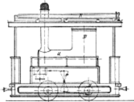
Č. 2610. Schema lokomotivy pro dráhy pouliční.
