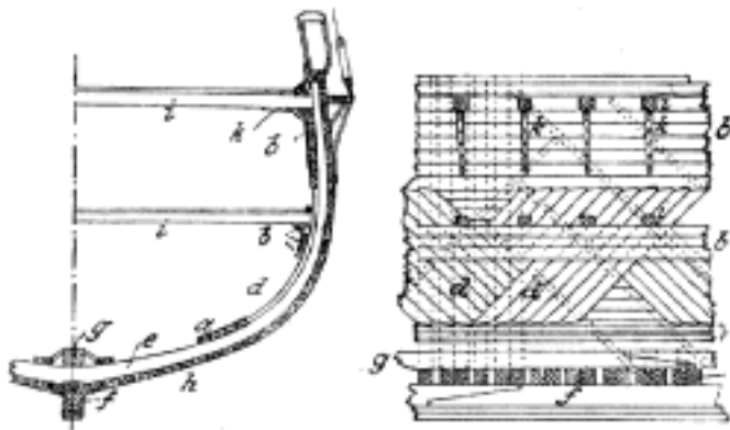
Č. 2579. a 2580. a podélné spjrní žeber, b podporné trámce podpalubních nosičů, d diagonální ztužení vnitřní, e příčná žebra, f kýl, g kýl vnitřní, h vnější stěna lodí, i trámce podpalubní, k úhlová železa k podpoře trámců podpalubních.
