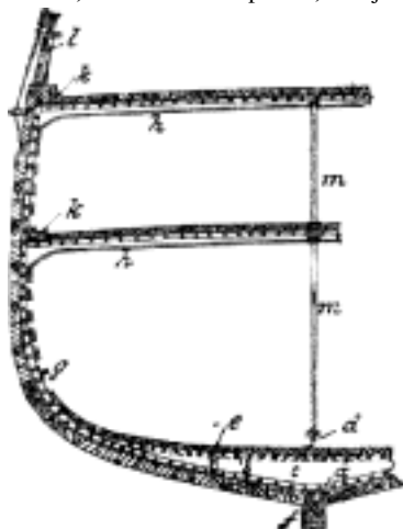
Č. 2582. a vnější úhelník žebra, b vnitřní úhelník žebra, c plech úhelníky spojující, d vnitřní kýl střední, e postranní kýl, f hlavní kýl, g úhelníky spojující žebra, h nosníky podpalubní, k plech vířící nosníky, l zábradlí, m podpory palub.
