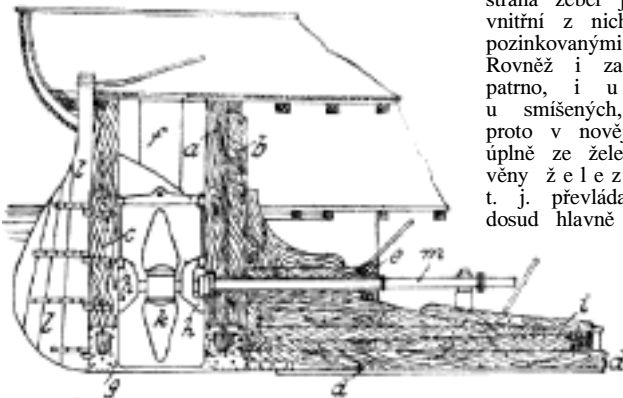
Č. 2578. a zadní stěven, b vnitřní stěven, c stěven pro kormidlo, d kýl, e trám se zacpávkou, f prohlubeň pro šroub, g železná spojení stěvenů, h stolice pro hřídel, i vnitřní kýl, k šroub, l kormidlo, m hřídel šroubový.
