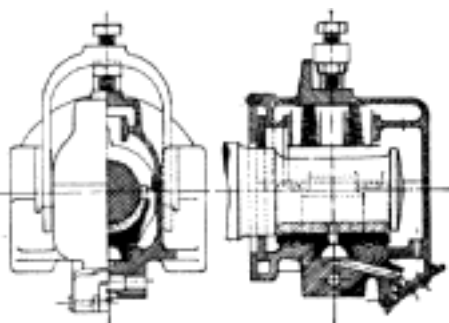
Č. 2629. Ložisko vozů železničních.
