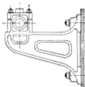
Č. 2624. Ložisko konsolové.
