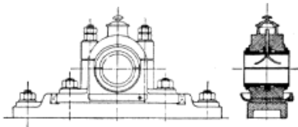
Č. 2621. Ložisko stojaté normální.
