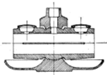
Č. 2627. Ložisko stojaté Sellersovo.
