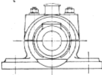
Č. 2627. Ložisko stojaté Sellersovo.
