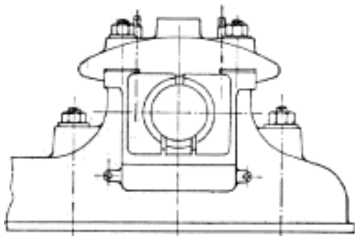
Č. 2623. Ložisko klíkové s trojdielnou pávní.
