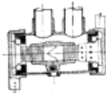
Č. 2628. Ložisko kuličkové.
