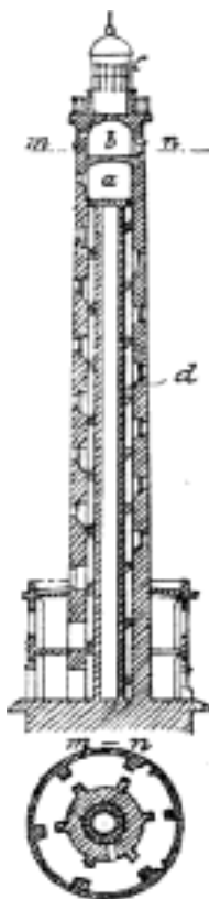
Č. 2655. Maják (průřez). a obydlí strážce, b zásobárna paliva, c osvětlovací přístroj, d točité schody.
