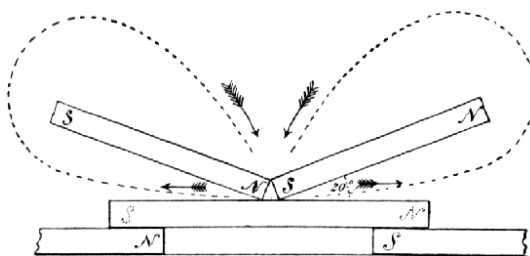
Č. 2644. Magnetisace jednoduchým tahem odděleným.
