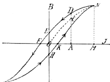
Č. 2646. Magnetická hysterese.
