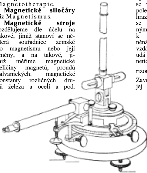
Č. 2647. Magnetický theodolit Lamontův.
