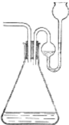
Č. 2670. Welterova ochranná trubice.
