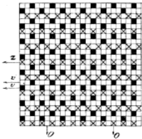
Č. 2673. Vatba pro hladký mašestr.
