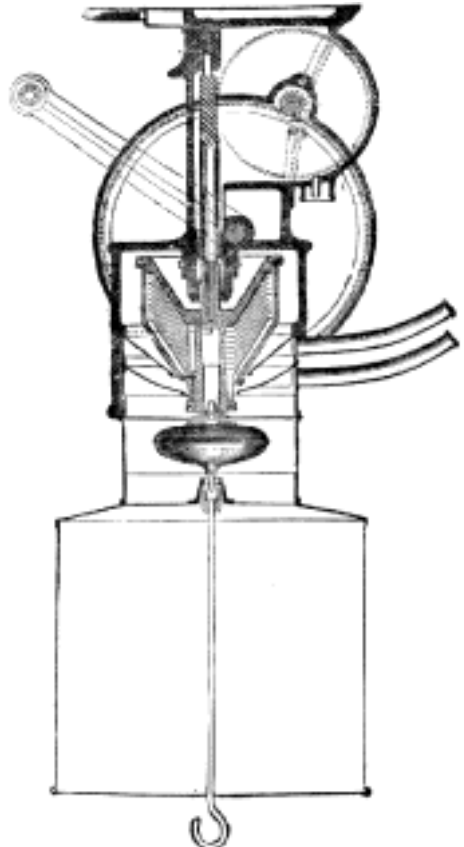
Č. 2699. Ruční odstřediv v průřezu.
