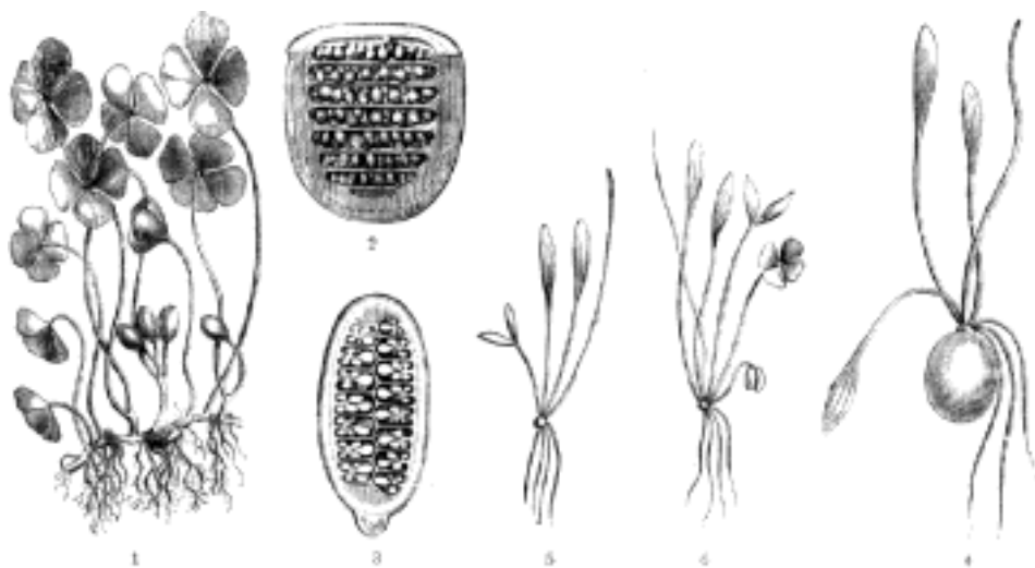
C. 2694. Marsilia . 1. Rostlina celá. - 2. a 3. Průřezy plodem na nichž viděti pouzdra a v nich oboje výtrusnice. - 4. Velkovýtrus zvětšený s kliční rostlinkou. - 5. a 6. Kliční rostlinky pokročilejší.
