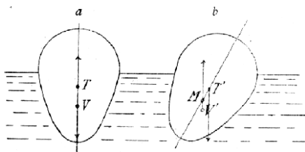
Č. 2745. Metacentrum polohy labilní.
