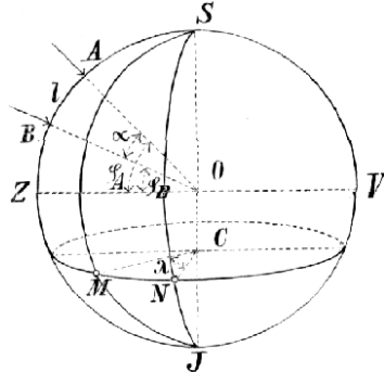
Č. 2726. Měření stupňové.
