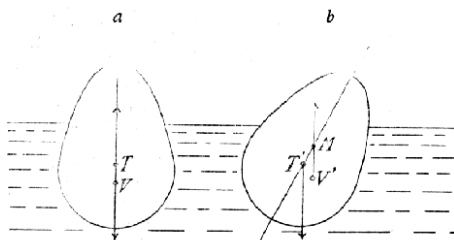
Č. 2746. Metacentrum polohy stabilní.
