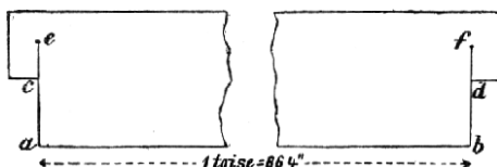
Č. 2727. Toise du Pérou.
