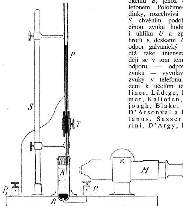
Č. 2750. Mikroelektrometr Lippmannův.
