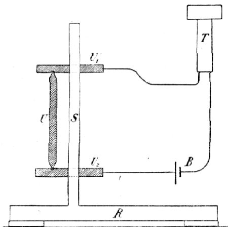
Č. 2751. Mikrofon.
