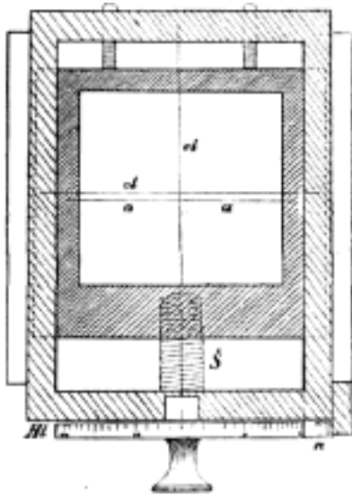
Č. 2753. Mikrometr vláknový (schema).
