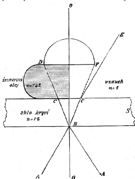
Č. 2759. Běh paprsků při immersii. OO osa drobnohledu; AB krajní paprsky osvětlující; BC tytéž v krycím skle S lomené; CD paprsek v oleji nelomený stíhá čočku DF; paprsek CE vve vzduchu lomený miji čočku DF.
