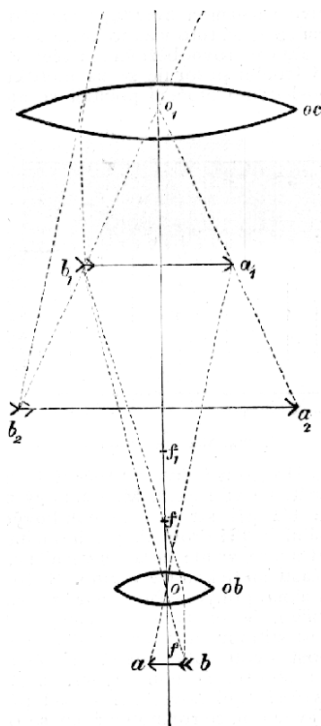
Č. 2757. Mikroskop složený. ob předmět; ob objektiv; f ohnisko objektivu; oc okulár; f1 ohnisko okuláru; a b1 skutečný obraz, vzniklý objektivem ob; a b2 zdánlivý obraz, pozorovaný okulárem oc; a o a1 o1 a2 směr paprsků světých.
