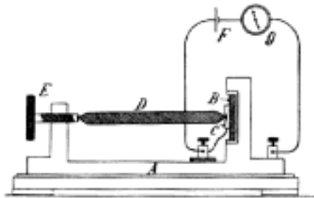
Č. 2760. Mikrotasimetr Edisonův.
