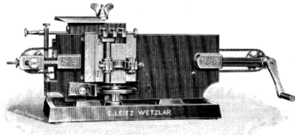
Č. 2761. Mikrotom.
