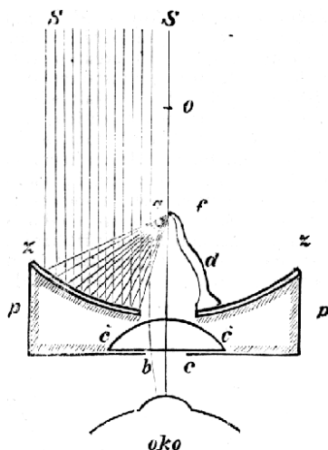
Č. 2758. Drobnohled Descartův. pp načeměné pouzdro; bc otvor, nad ním čočka čč; zz zrcadlo duté s otvorem uprostřed; d držák na předmět; f ohnisko a předmět.
