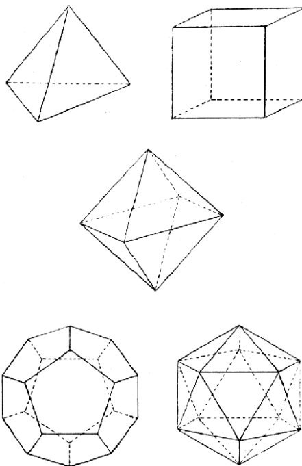
Č. vyobr. 2791. Čtyřstěn. Šestistěn. Osmistěn. Dvanáctstěn. Dvacitstěn.
