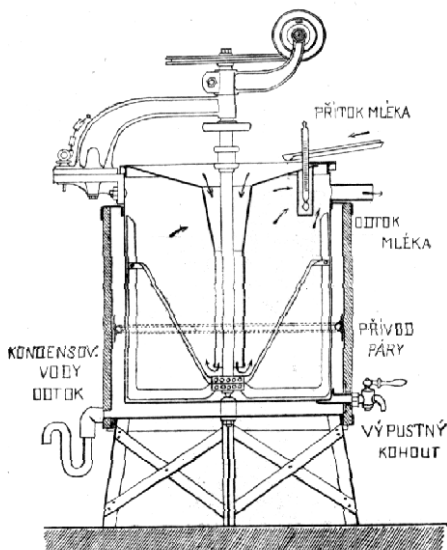
Č. 2783. Pasteur na mléko.
