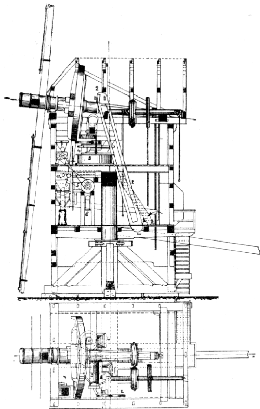
Č. 2786. Větrný mlýn německý.
