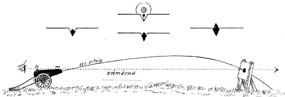
Míření jemnou neb nízkou muškou plnou muškou hrubou neb vasokou muškou h hledí, m muška. Č. vyobr. 2775.
