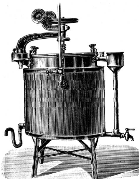
Č. 2783. Pasteur na mléko.
