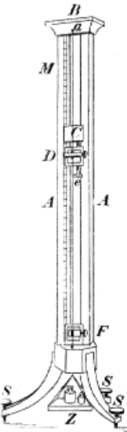
Č. 2813. Monochord Weberův.
