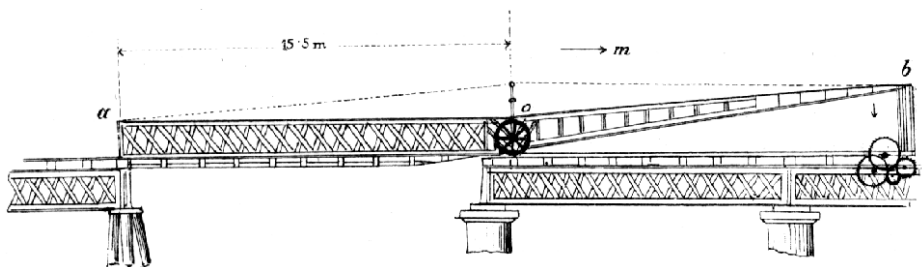
Č. 2830. Posuvný most na viaduktech v Barmouthu.
