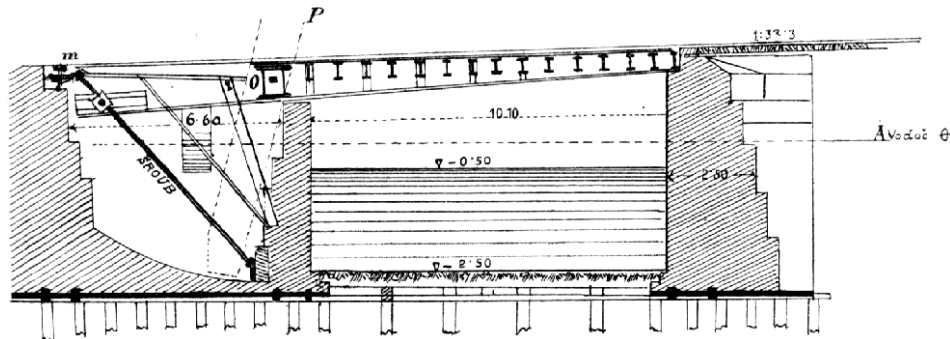
Č. 2833. Sklápěcí most v Amsterdamě.
