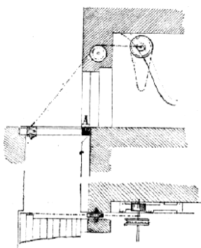
Č. 2832. Výtahový most dle Belidora.
