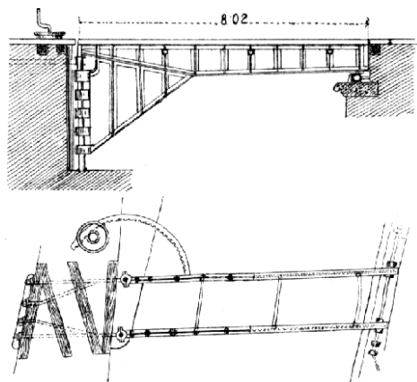
Č. 2835. Jestřábový most u Zwolle nizozemské provincie
