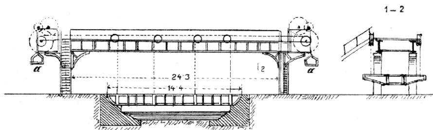
Č. 2831. Zdvíhací most u Rosières-aux-Salines.
