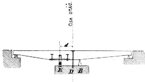
Č. 2834. Typ mostu otáčivého s osou u středu.
