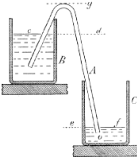
Č. 2863. Násoska ohnutá.
