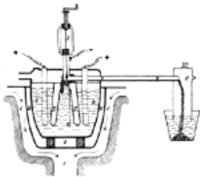
Č. 2865. Grabauův přístroj.
