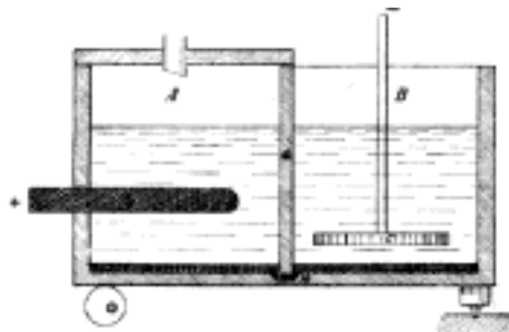
Č. 2866. Castnerův přístroj.
