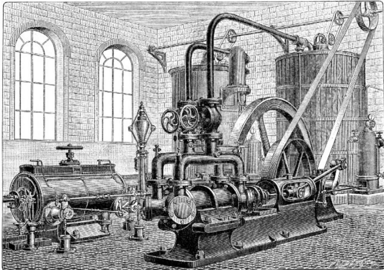
Chladicí stroj s bezvodým čpavkem, soustavy inž. Fixary-ho.
