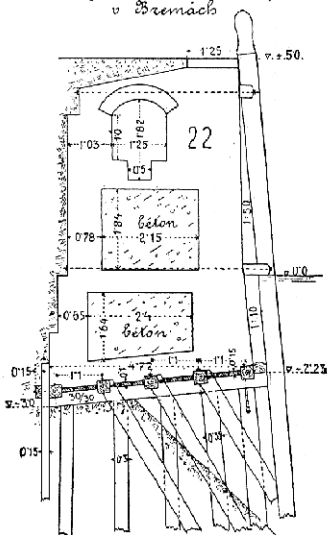
Rošt jablový přístavni zdi v Břeměch
