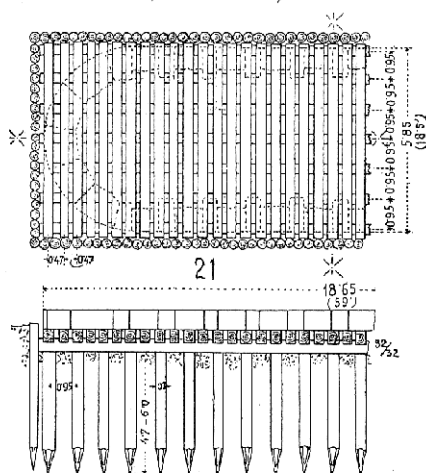
Rošt jehlový Františkova mostu celézovského v Praze
