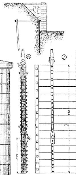
Uložení ošpice.
