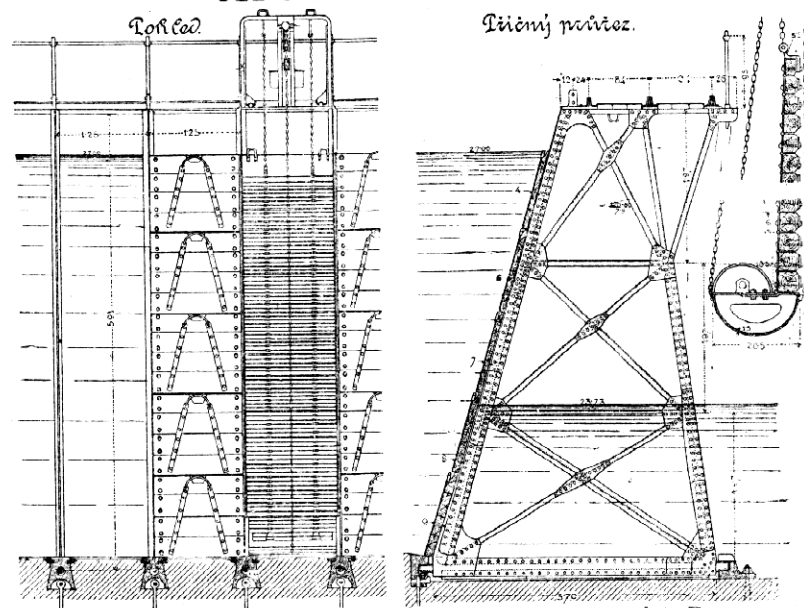
JEZ DESFONTAINES-ŮV NA MOHANU.
