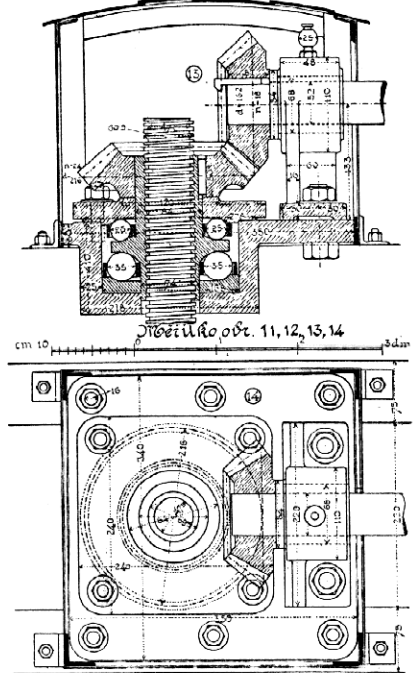
Lištník ku pohybu stavidel.
