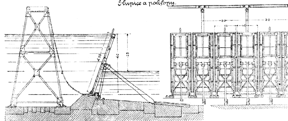
MULATIÈRSKÝ JEZ U LYONU
