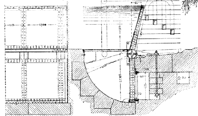
JEZ DESFONTAINES-ŮV NA MOHANU.
