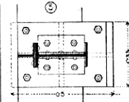
Uložení ošpice.
