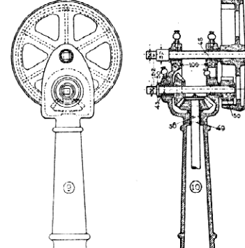
Lištník ku pohybu stavidel.
