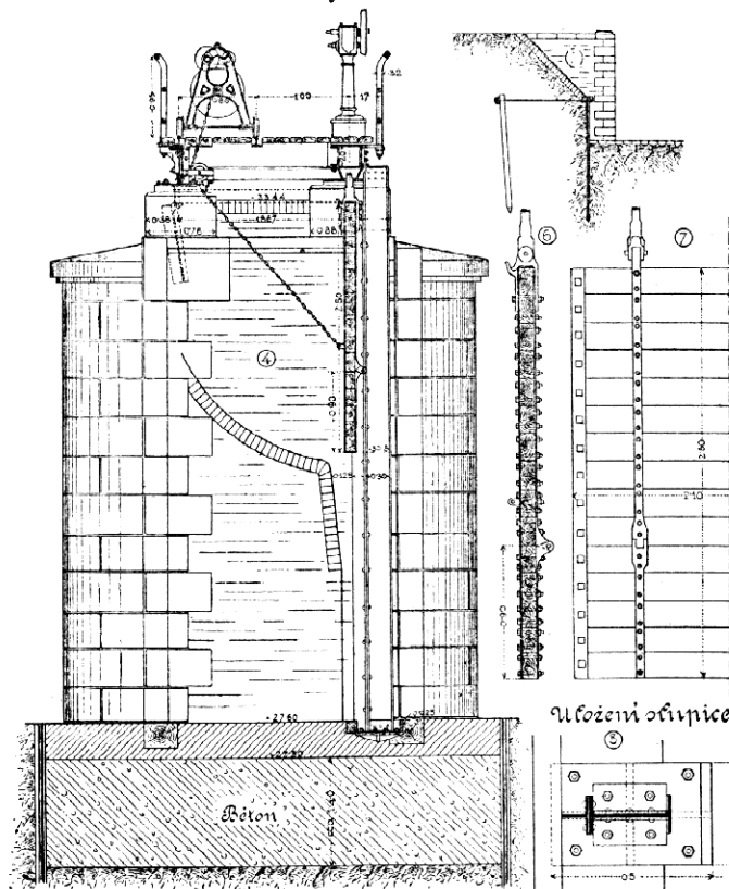
Řez a-b.
