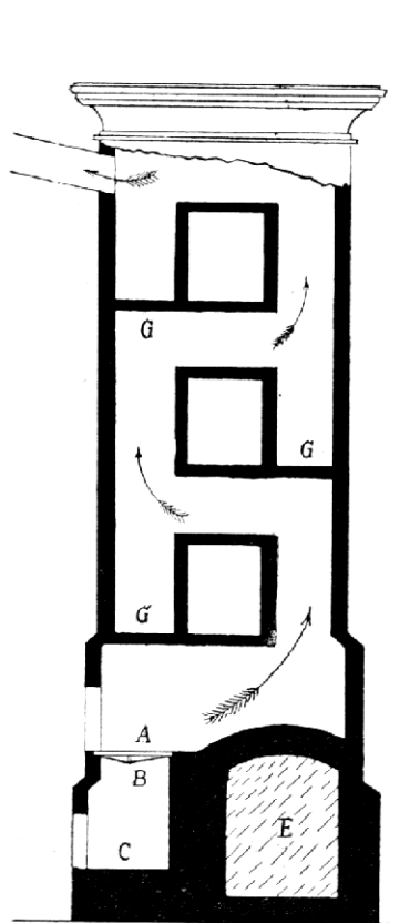
Kamna tahová (plzeňky).
