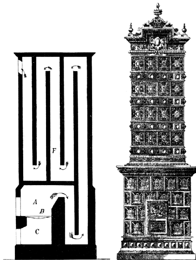
Kamna s hermetickým uzavřením.
