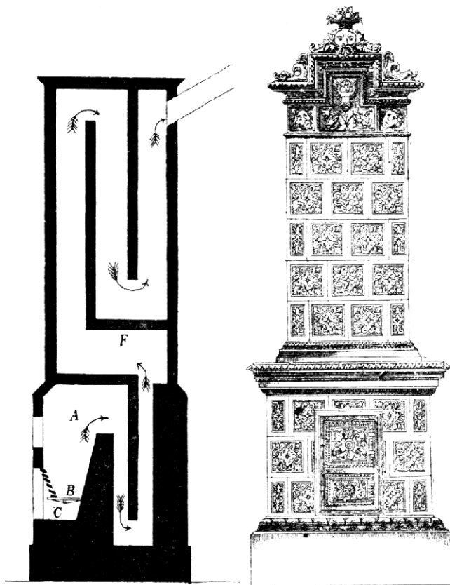
Kamna regulační s vyhříváním ze spodu.
