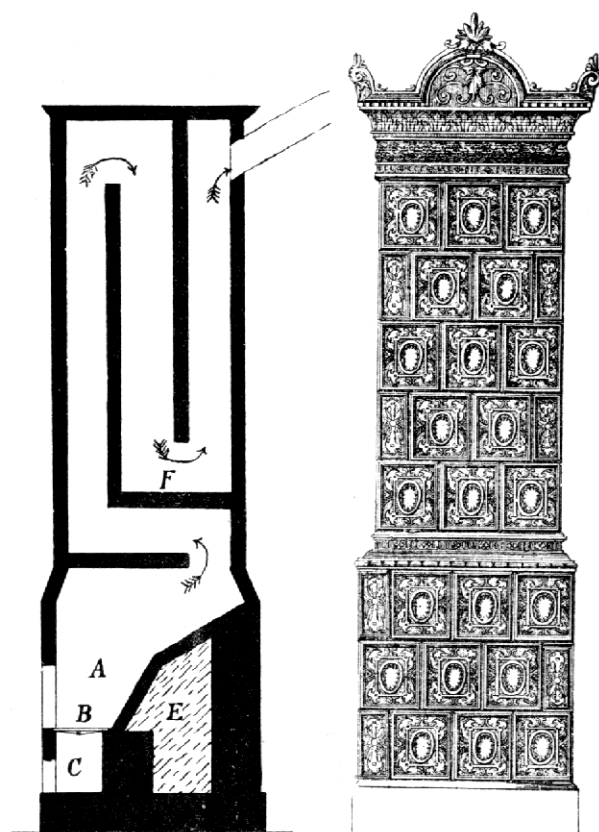
Kamna s tahy kolnými.
