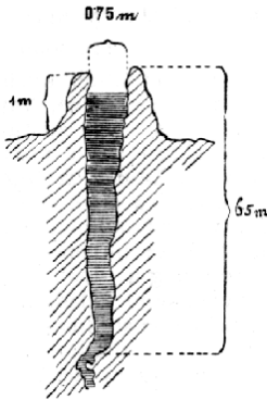
Č. 1552. Profil geysiru Bee-hive.
