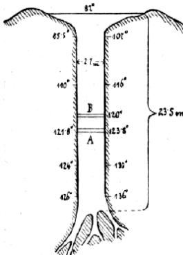
Č. 1553. Schem. profil Velkého Geysiru na Islandě.
