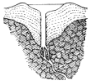
Č. 1554. Profil Velkého Geysiru, vysvětlující vznik studny, kužele a pánve.
