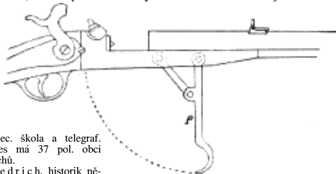
Č. 1555. Ghayevova ručnice otevřena.
