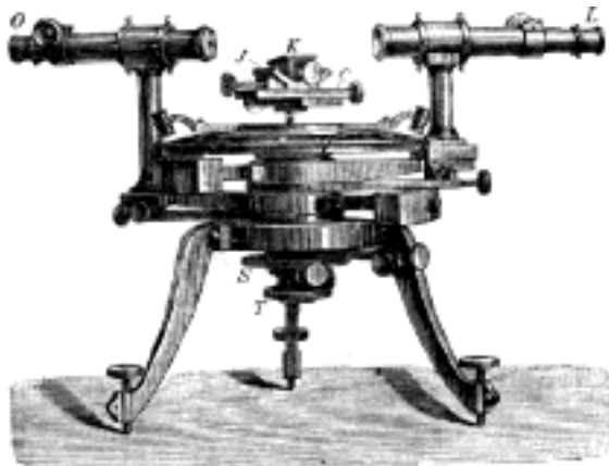
Č. 1574. Odrazný goniometr dle Babineta. V kruh dělený, S dutá osa, T vnitřní osa, C přístroj centrační, J přístroj justační, K nosič krystalu, L kollimátor, O dalekohled pozorovací.
