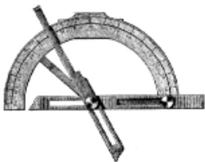
Č. 1571. Goniometr příložený nebo Carangeotův.
