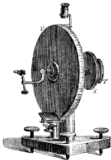
Č. 1572. Odraslý goniometr Wollastonův. V kruh dělený, S dutá osa, T vnitřní osa.
