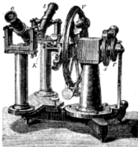
Č. 1573. Odraslý goniometr dle Mitscherliche. V kruh dělený, S dutá osa, T vnitřní osa, C přístroj centrační, K nosič krystalu, L kollimator, O dalekohled pozorovací.
