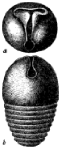
Č. 1569. Gomphoceras Bohemicum Barr.: a pohled s hory, b se strany břišní.
