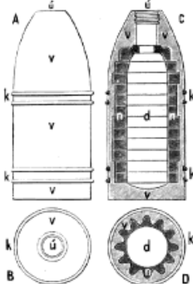
Č. 1593. Granát ogivální rázu nového. A) pohled vnější se strany, B) pohled vnější shora, C) průřez se strany, D) průřez shora.
