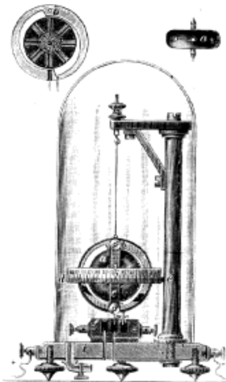
Č. 1615. Elektrický gyroskop Trouvého.
