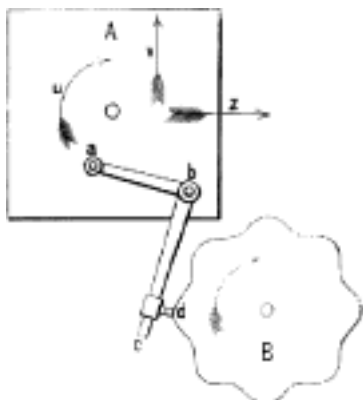
Č. 1601. Schema stroje guillochovacího.
