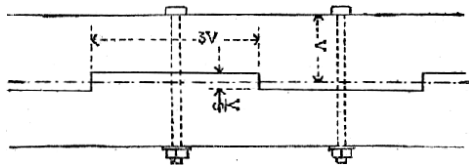
Č. 1640. Hákování.
