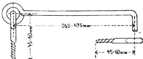
Č. 1638. Hák rozpěrací.
