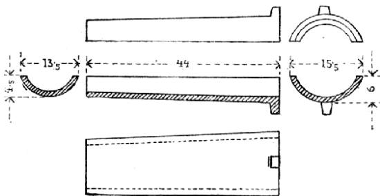
Č. 1639. Hák (taška).
