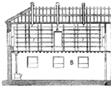
Č. 1669. Magnanerie (řez podélný a příčný).
